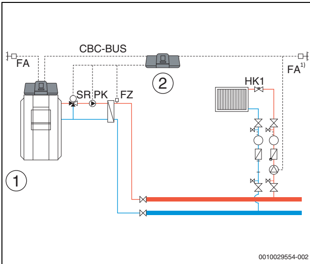
Bild 33 Variante 1: Unterstation mit Vormischfunktion, Kompensation Wärmeverluste über FZ, Lastbegrenzung
