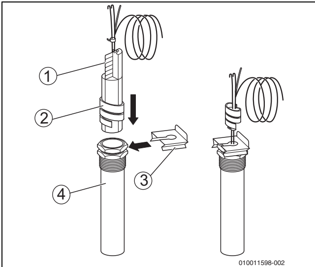
Bild 7 Kunststoffspirale in Tauchhülse einsetzen@@
