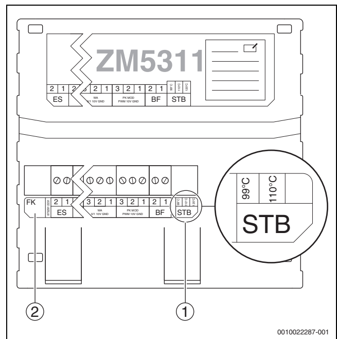
Bild 24 Elektronischer Sicherheitstemperaturbegrenzer beim ZM5311
