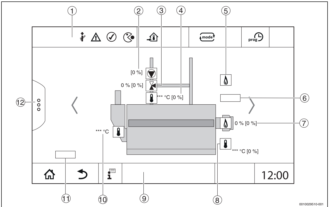
Bild 12 Anzeige Wärmeerzeugung (Beispiel)
