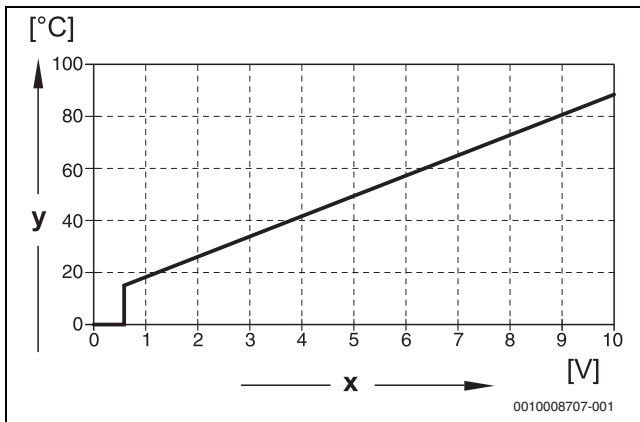
Bild 28 0...10-V-Eingang Temp.
