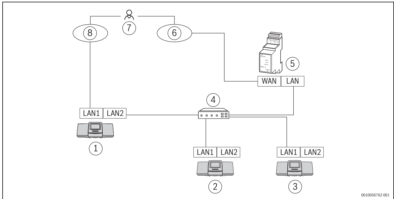
Bild 47 Beispiel einer Regelgeräteanbindung mit Fernzugriff und Gebäudeleittechnik
