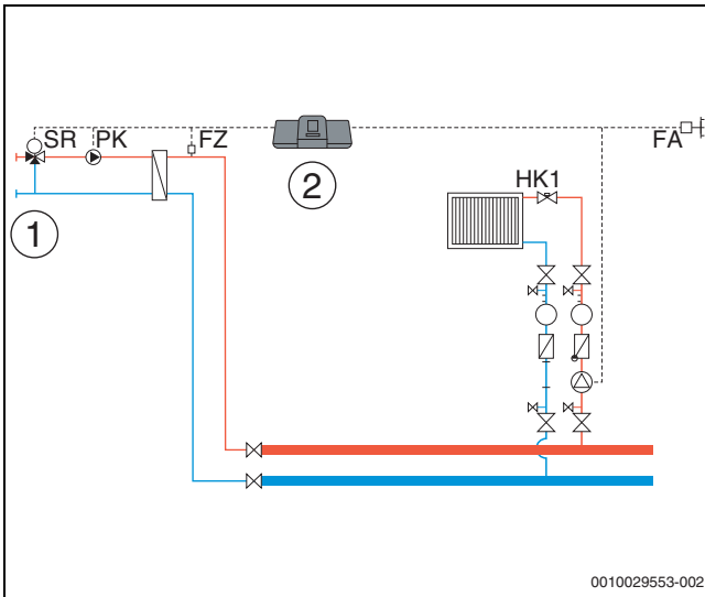
Bild 32 Variante 3: Fremde Wärmequelle ohne Zubringerpumpe, Lastbegrenzung, Vormischfunktion, Kompensation Wärmeverluste über FZ
