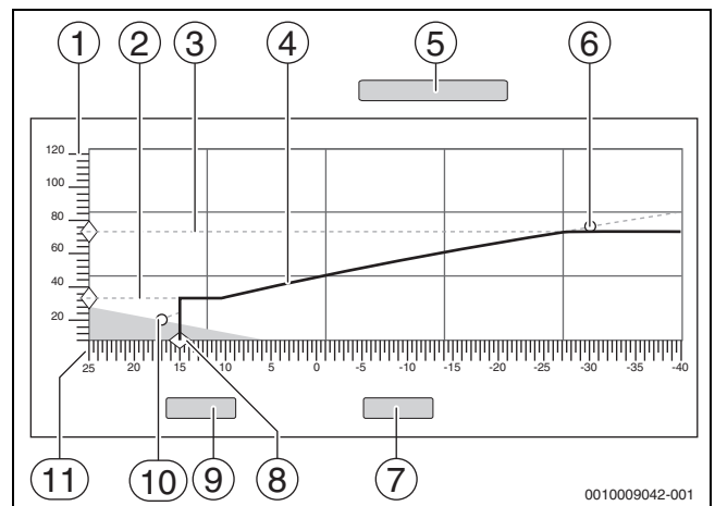
Bild 43 Heizkurve
