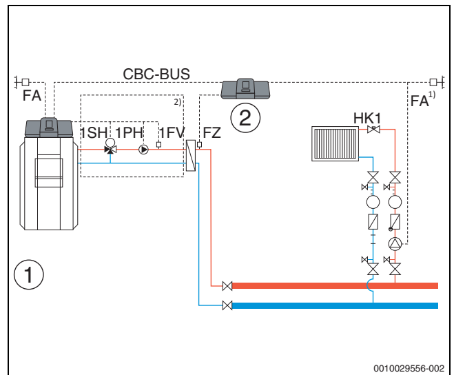
Bild 35 Variante 3: Unterstation mit Vormischfunktion, Kompensation Wärmeverluste über FZ, Lastbegrenzung und Heizbetrieb bei Kommunikationsverlust
