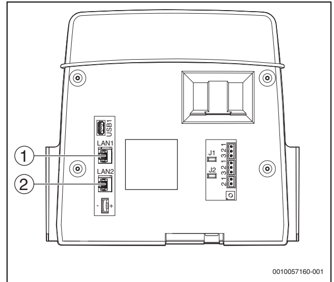
Bild 45 Anschluss für LAN1 und LAN2
