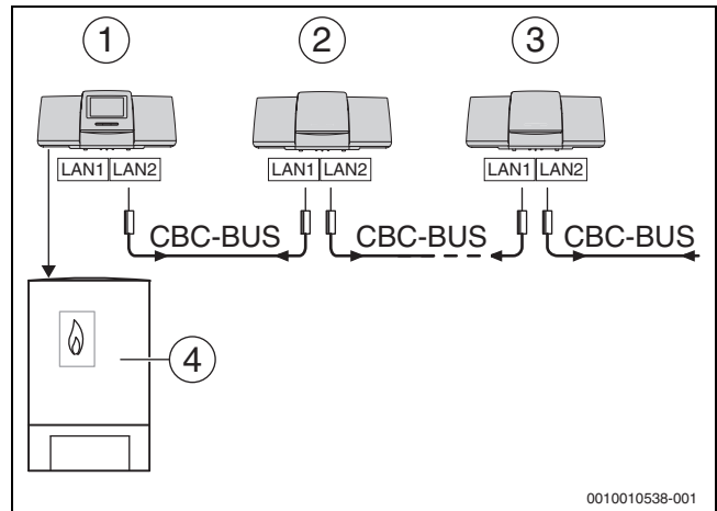
Bild 46 Beispiel einer Regelgeräteanbindung mit mehreren Regelgeräten
