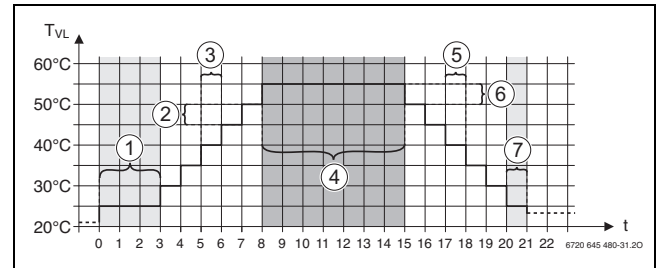
Bild 44 Estrichtrocknung
