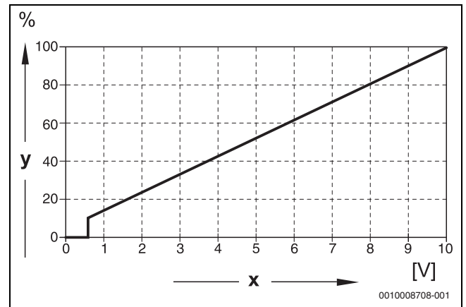
Bild 29 0...10-V-Eingang Leistung
