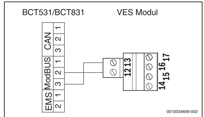
Bild 37 Anschluss des Regelgeräts an das VES Modul
