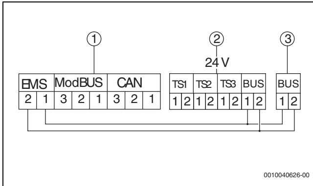
Bild 5 Elektrischer Anschluss
