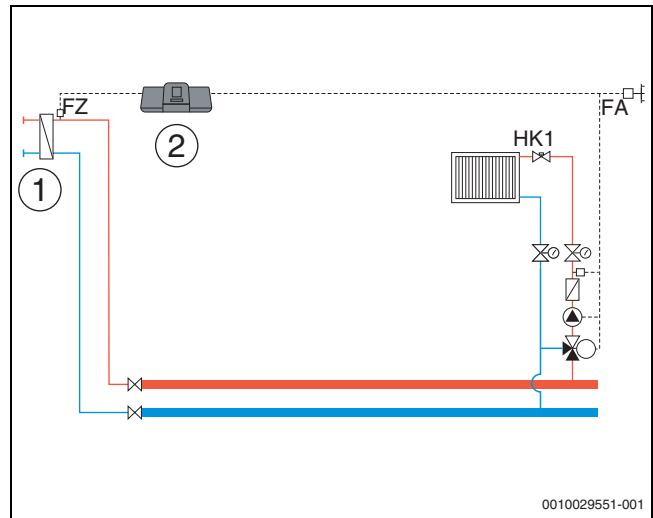
Bild 30 Variante 1: Fremde Wärmequelle mit Zubringerpumpe, Lastbegrenzung und Kompensation Wärmeverluste über FZ
