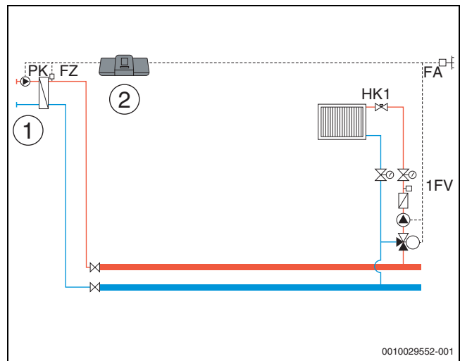
Bild 31 Variante 2: Fremde Wärmequelle ohne Zubringerpumpe, Lastbegrenzung und Kompensation Wärmeverluste über FZ
