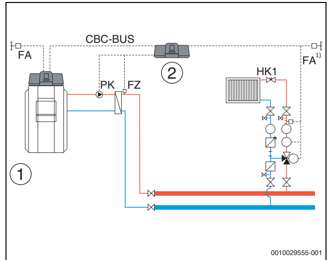
Bild 34 Variante 2: Unterstation mit Kompensation Wärmeverluste über FZ, Lastbegrenzung
