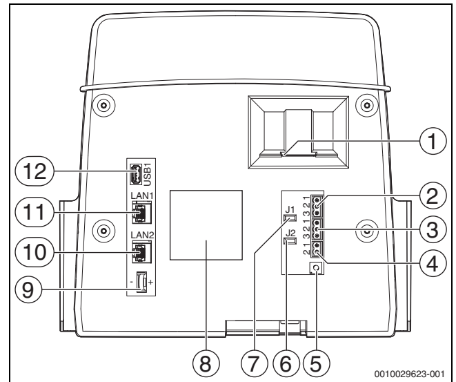
Bild 23 Rückseite Bedieneinheit
