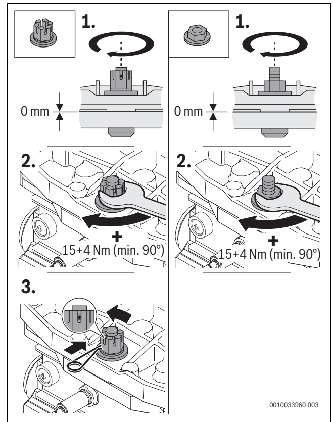
Bild 12 Mutter am Brennerdeckel festziehen
