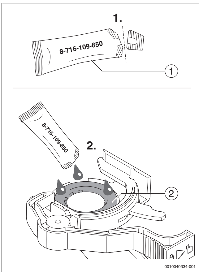
Bild 18 Dichtung fetten
