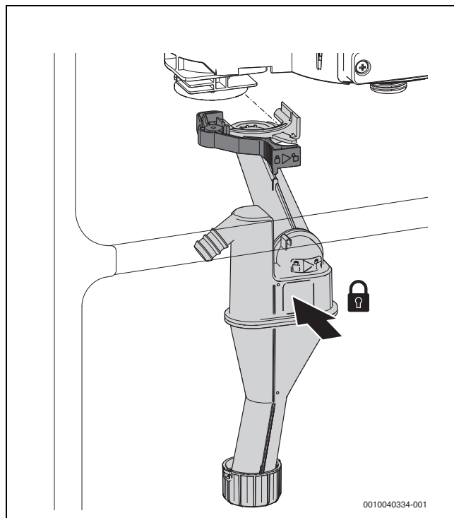
Bild 19 Kondensatsiphon einsetzen
