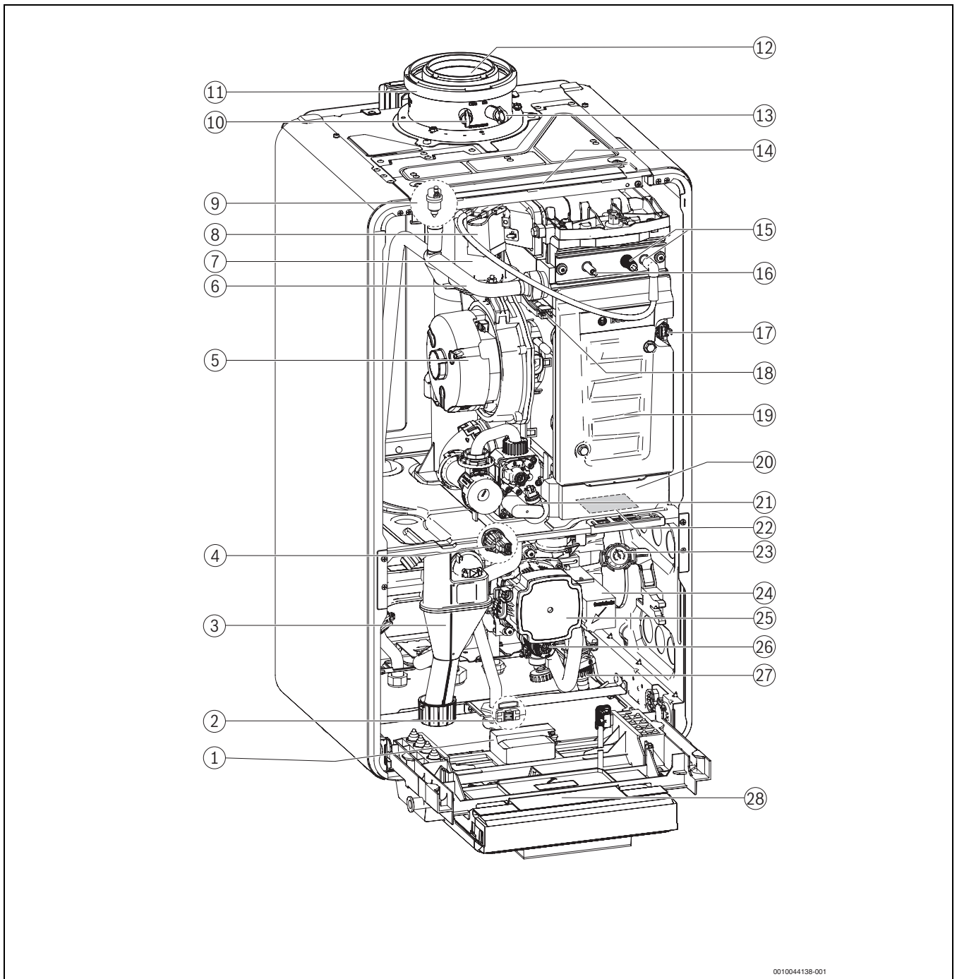
Bild 2 Produktübersicht Speichergerät
