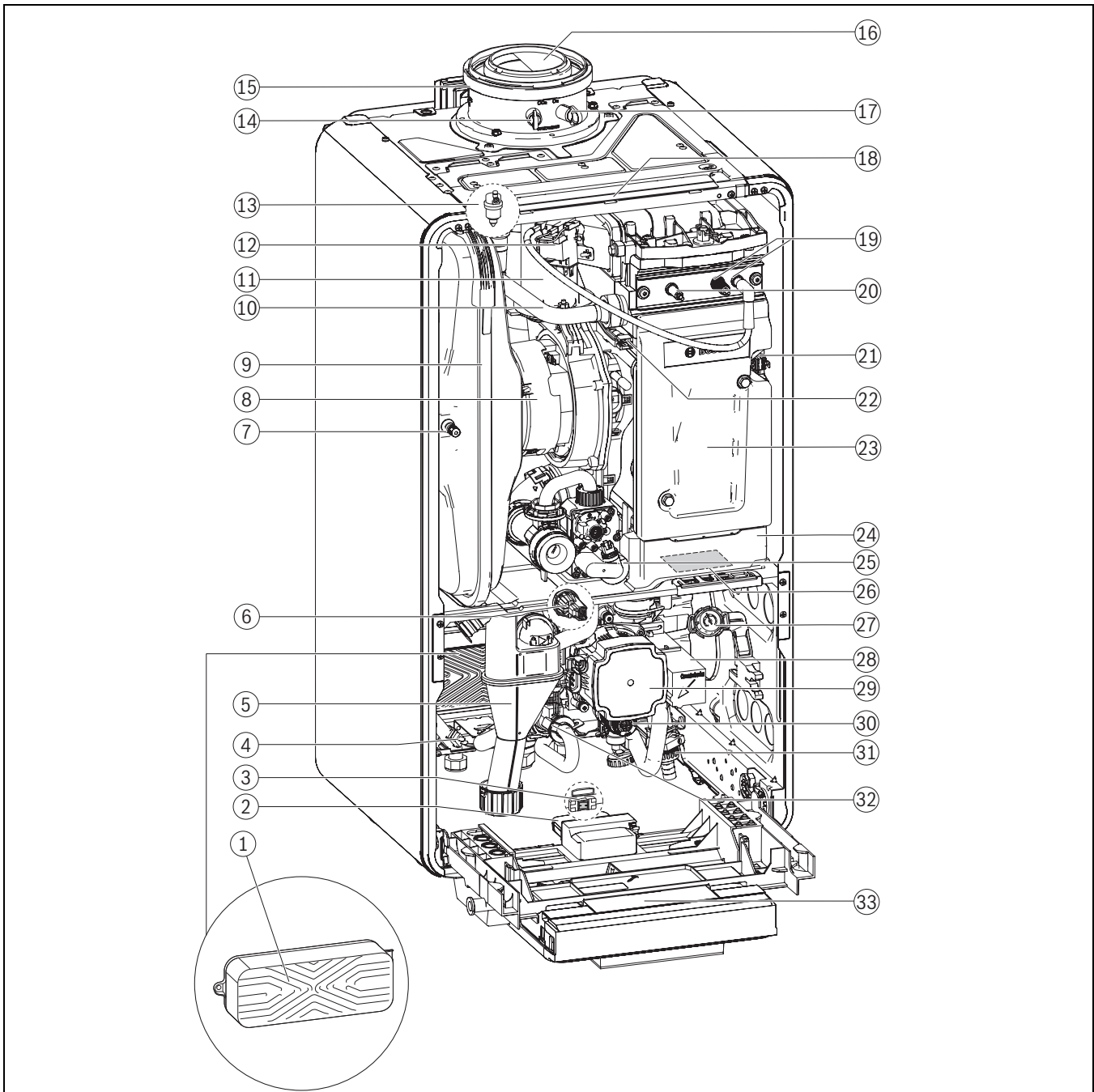
Bild 1 Produktübersicht Kombigerät
