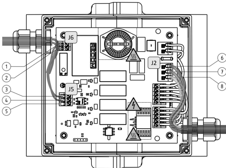
Ilustracja 1: Płytkę z przykładowymi przewodami przyłączeniowymi (możliwe różnice w wyposażeniu płytki)
