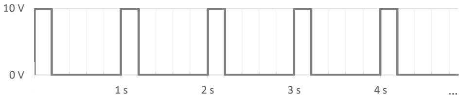
Signál PWM: Délka periody 1 s; délka pulzu 200 ms
