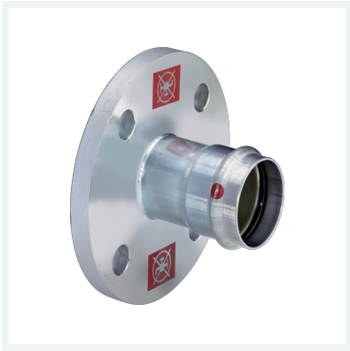
Prestabo-Flanschübergang mit SC-Contur Modell 1159.1 Artikel 642 389
