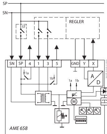
AME 658: Verdrahtung für die modulierende Regelung
