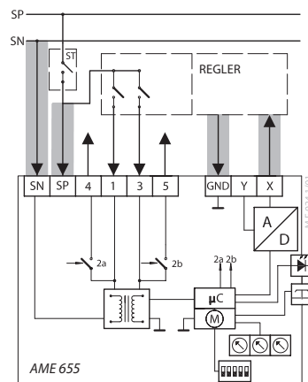
Optional: AME 655 als 3-Punkt-Ausführung angeschlossen
