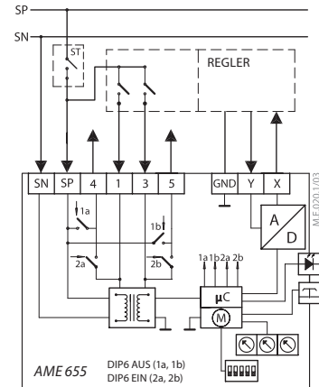
AME 655: Verdrahtung für die modulierende Regelung
