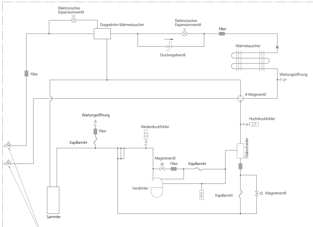
Absperrventil (mit Wartungsöffnung an bauseitiger Rohrleitungsseite, ø 6,4 mm Bördelverbindung)
