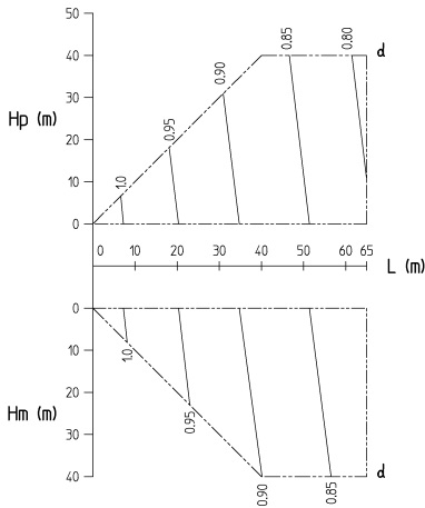
Änderungsrate der Kühlleistung von ERQ100, ERQ125
