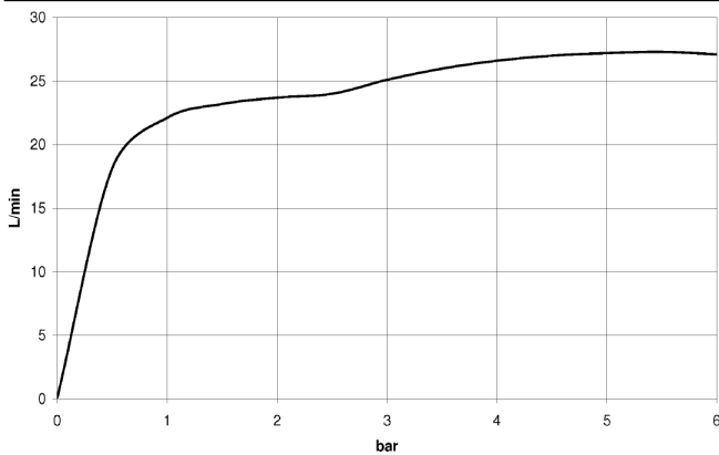
Durchflussdiagramm
