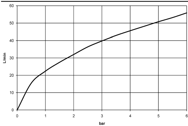
Durchflussdiagramm
