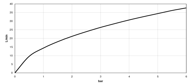
Durchflussdiagramm
