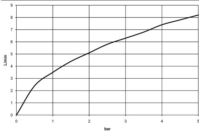
Durchflusssdiagramm
