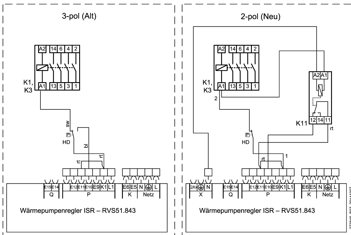
Abb. 1: Schaltplan
