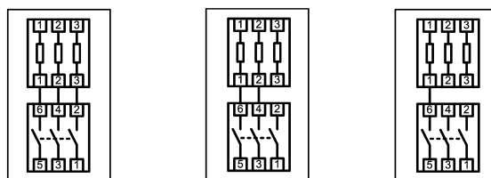
Abb. 1: Anschluss Elektroheizeinsatz K26
