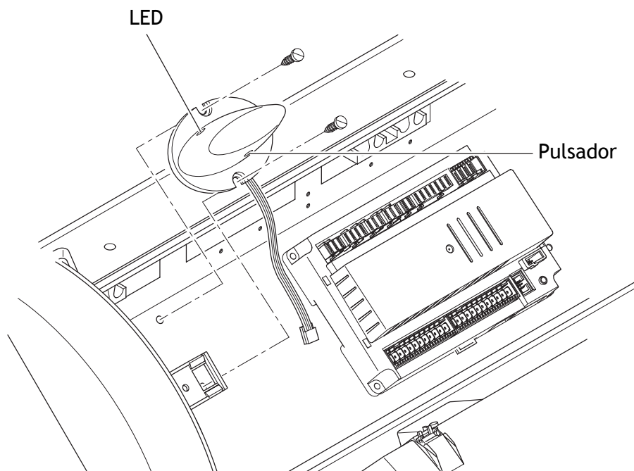
Fig. 3: Montaje del radioreceptor FEK
