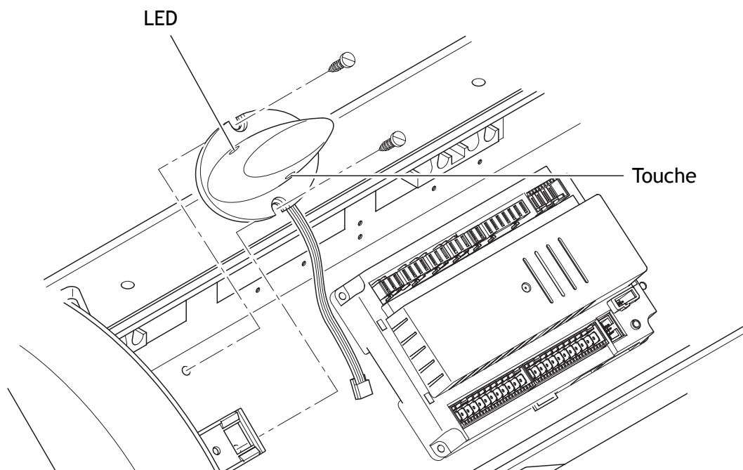
Fig. 3: Montage du récepteur radio FEK
