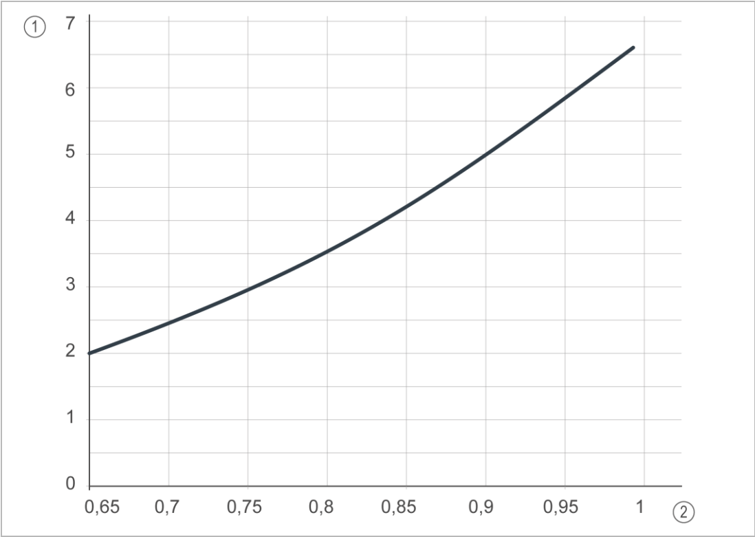
Durchfluss in Abhängigkeit von SSK_{254nm} / \tau (10)
