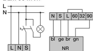
DL 32 m³/h BLm 90 m³/h
