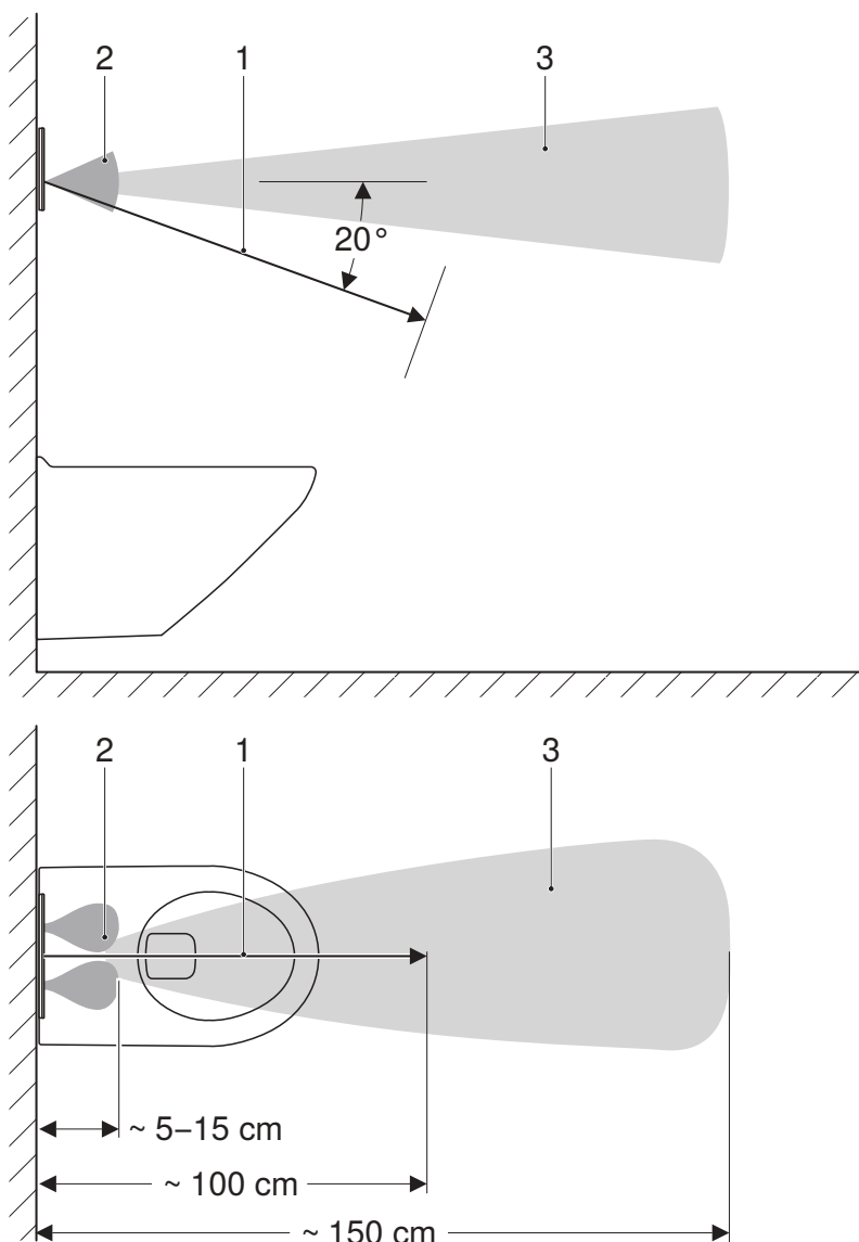
Billede 1: Registreringsområder
