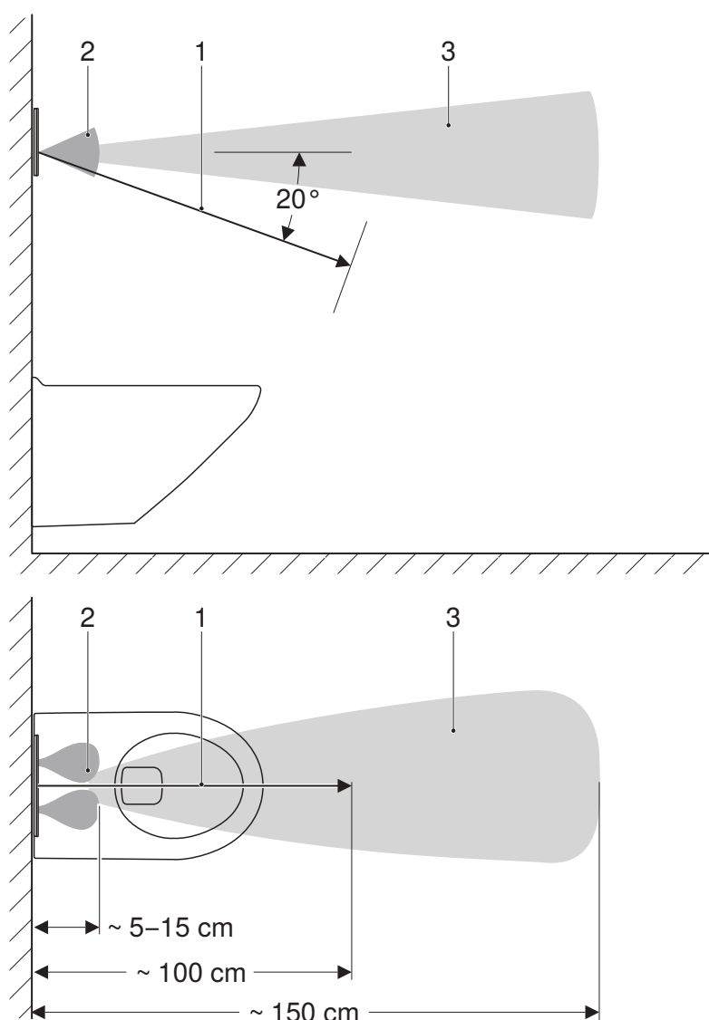
Obrázek 1: Snímací rozsahy
