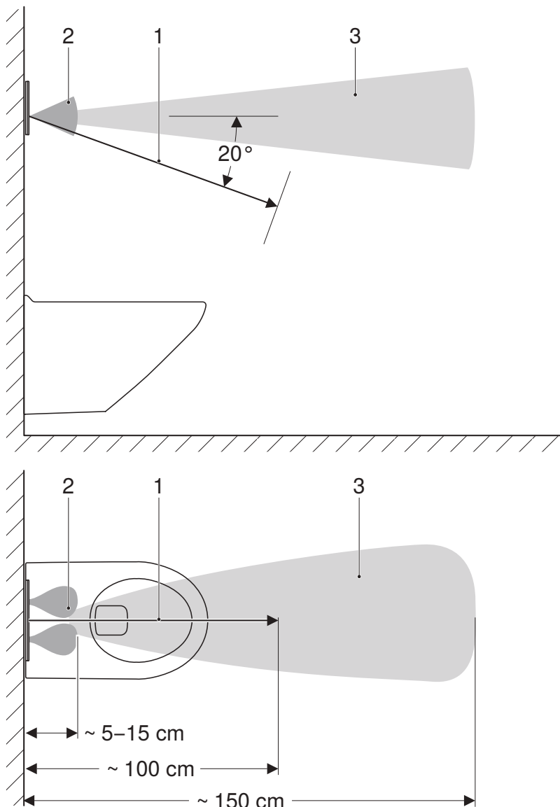
Mynd 1: Skynjunarsvið
