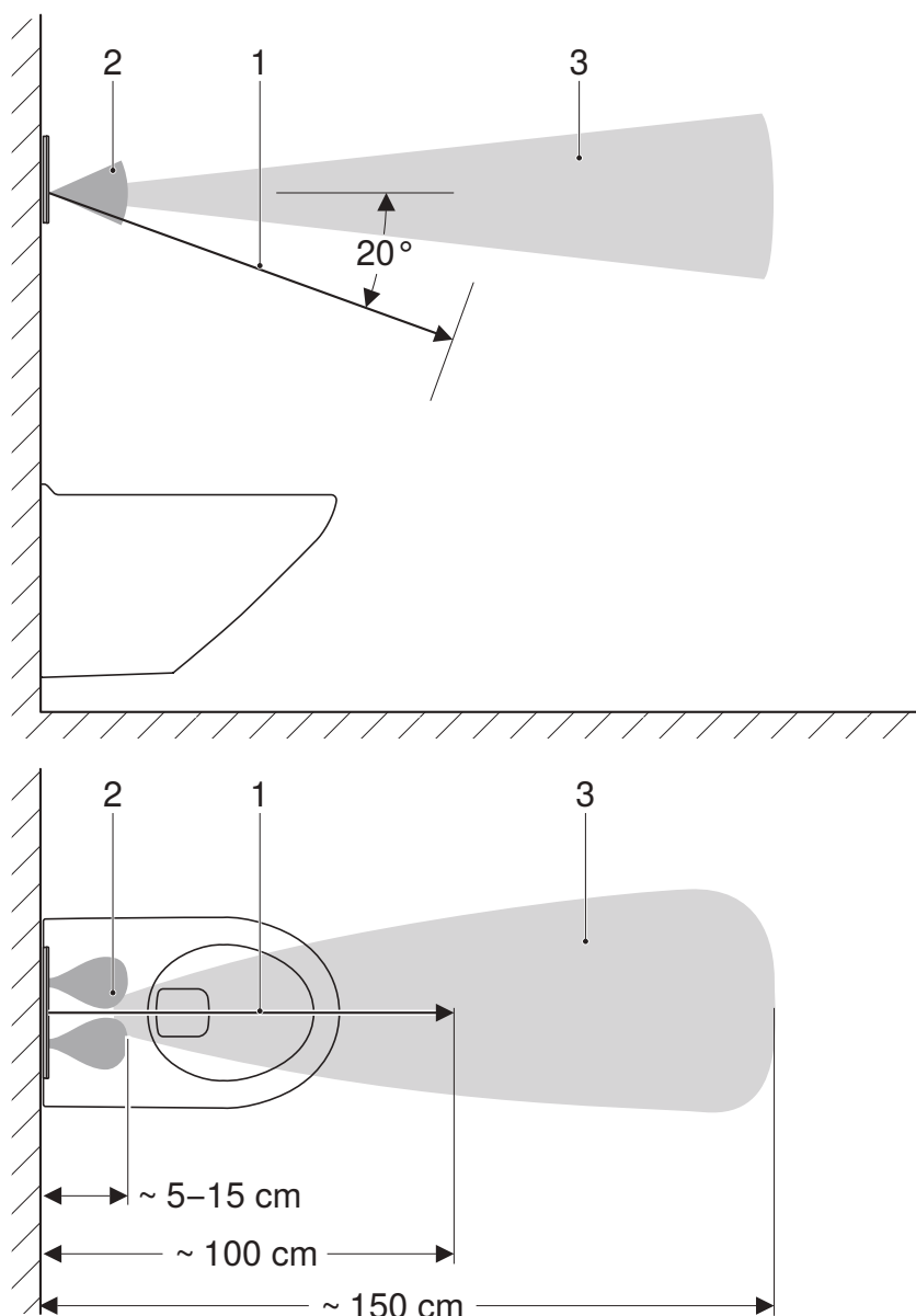
Slika 1: Područja detekcije
