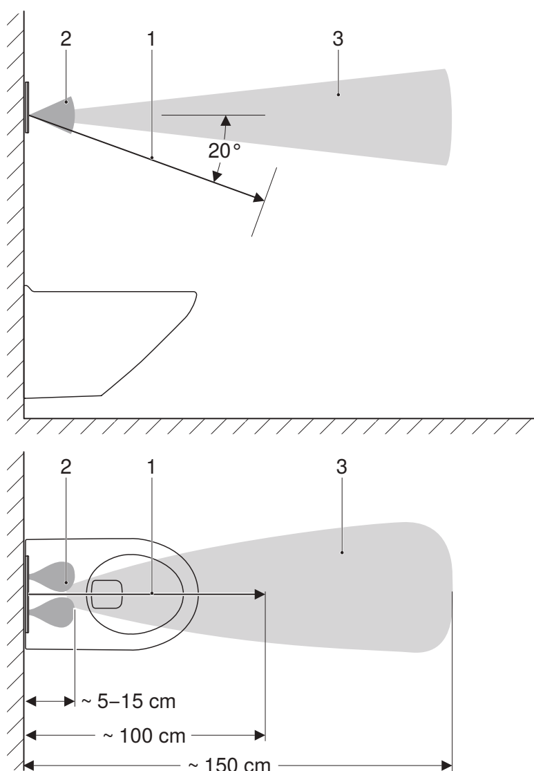
Obrázok 1: Detekčné oblasti
