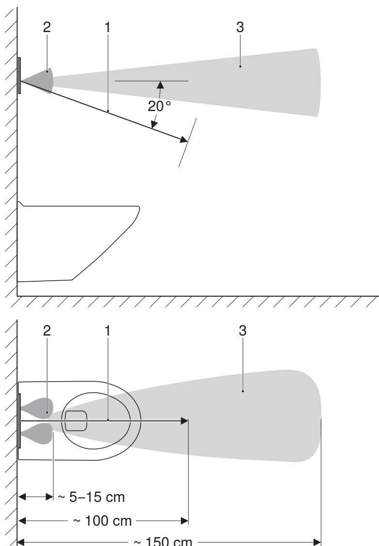
Εικόνα 1: Γωνίες ανίχνευσης
