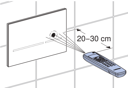
插图 2: 用 Geberit 服务遥控器进行操作 Geberit 服务遥控器提供了下列功能和设置：
