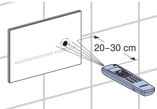
Obrázek 2: Obsluha pomocí servisního dálkového ovládání Geberit
