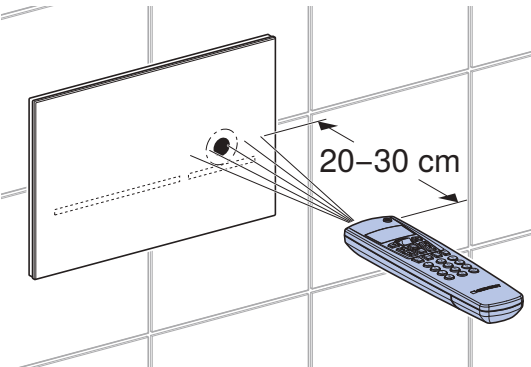
Bilde 2: Betjening med Geberit Service-mobilen Med Geberit Service-mobilen har du følgende funksjoner og innstillinger til rådighet:
