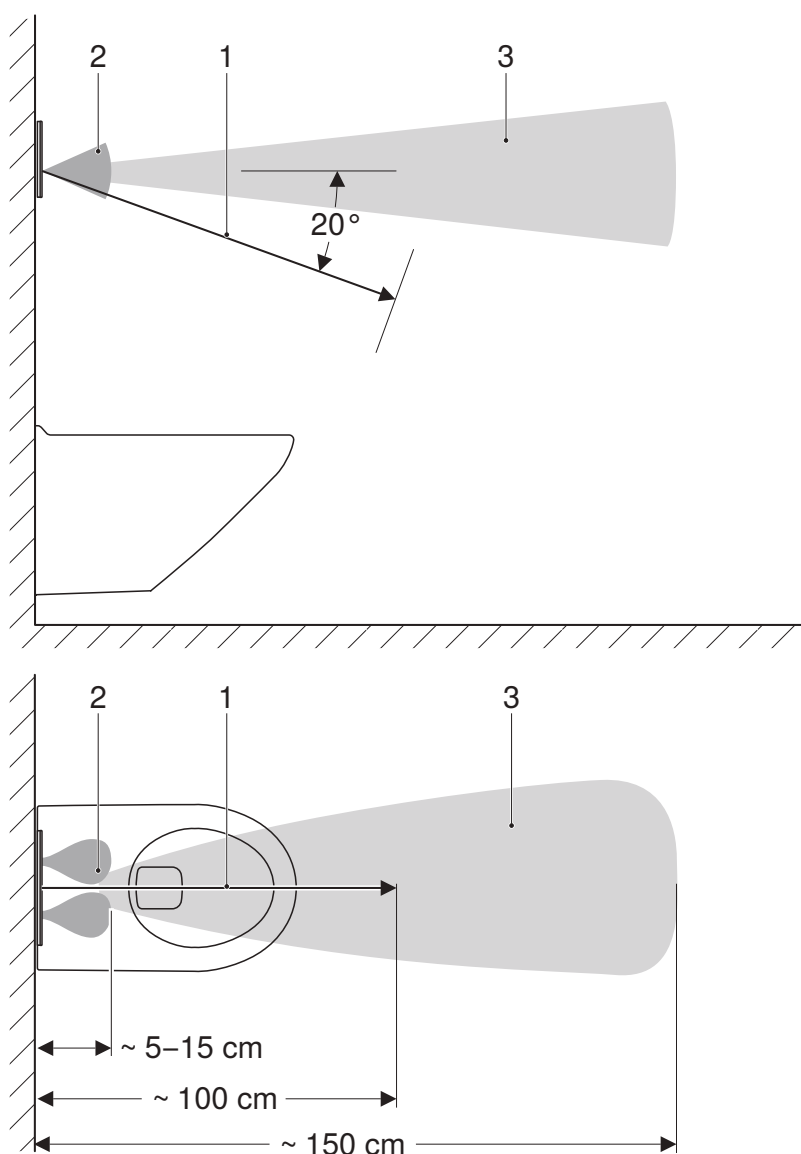
Рисунок 1: Диапазоны распознавания
