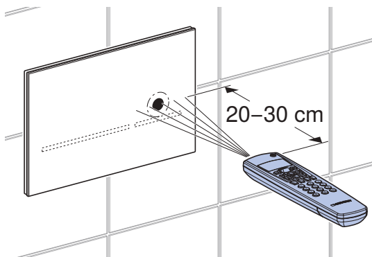
Илустрација 2: Ракување со сервисниот мобилен телефон на Geberit
