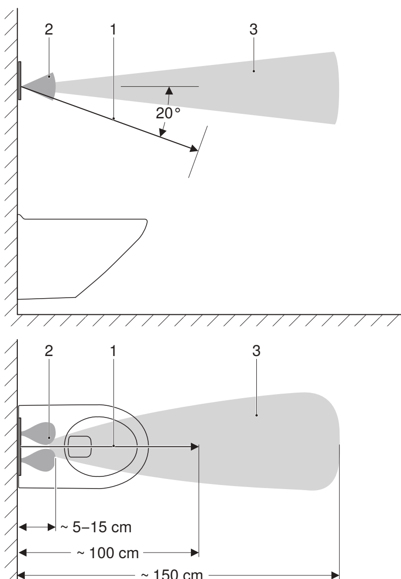
Bilde 1: Registreringsområder
