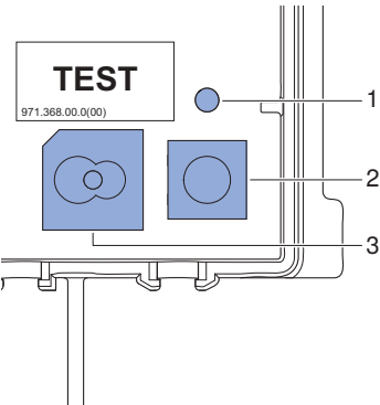
Afbeelding 2: Weergaven en bedienelementen op de besturingseenheid
