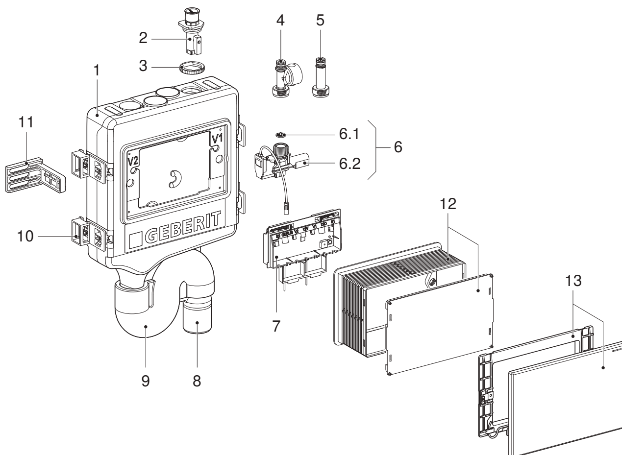
Illustration 1: Rîņages forcés hygiéniques Geberit HS30 et HS50
