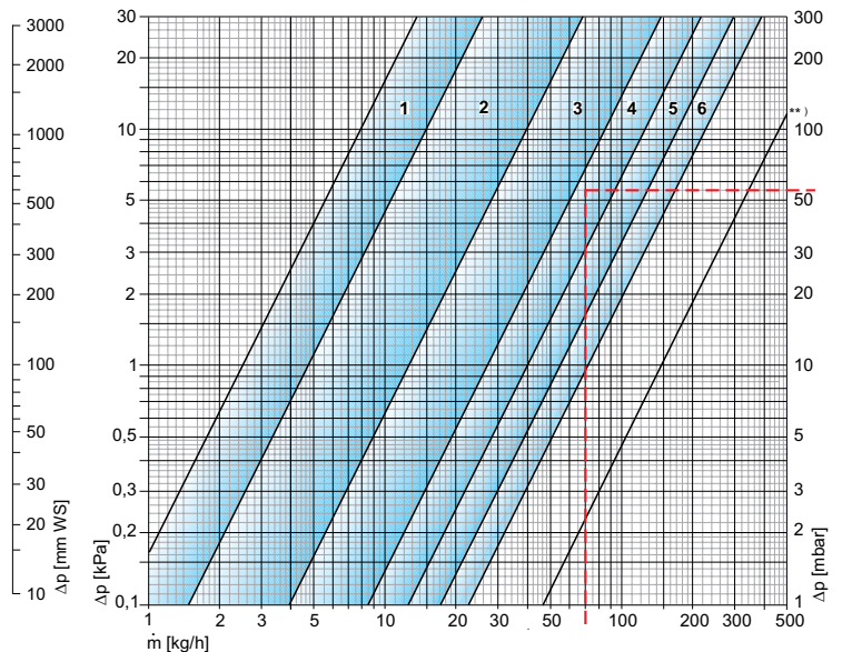
Thermostat-Oberteil VHV mit 6 Einstellbereichen
