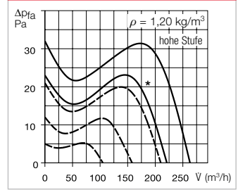
* niedrige Stufe --- Beispielhafte Leistungsstufen der 0-10 V Type bei stufenloser Regelung
