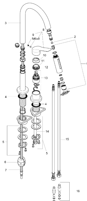
部品リスト
