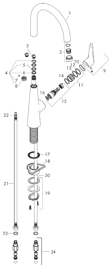
製品分解図
