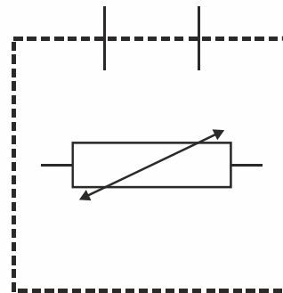
Abb. 2. SF00, SF10 und SF20 Verdrahtung
