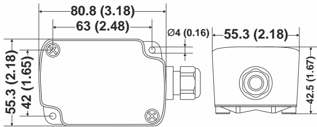
Abb. 1. Abmessungen des SF00/SF10/SF20 in mm (Inch)
