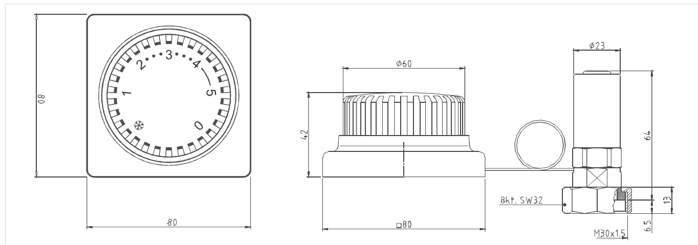
Abb. 1 Baumaße
