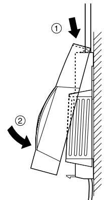
Afbeelding 4: Deksel op de behuizing plaatsen
