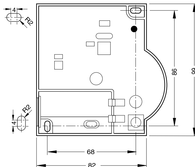
Figur 3: Bore-skabelon (angivelser i mm)
