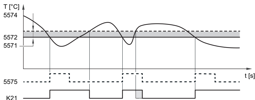
Abb.30 Überwachung Temperaturunterschreitung
