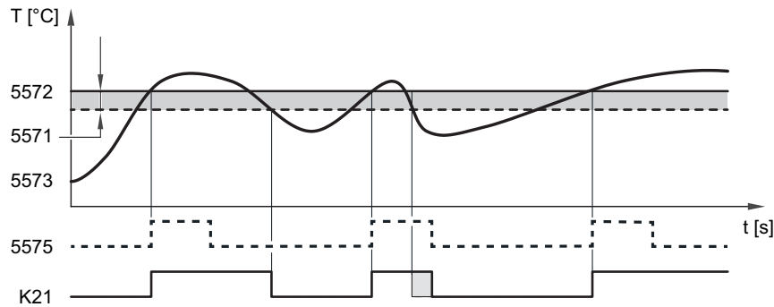
Abb.29 Überwachung Temperaturüberschreitung
