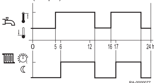
Abb.24 Freigabe in Abhängigkeit von den Zeitprogrammen der Heizkreise (Beispiel)
