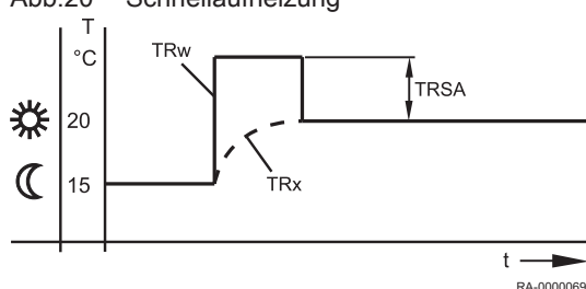
Abb.20 Schnellaufheizung
