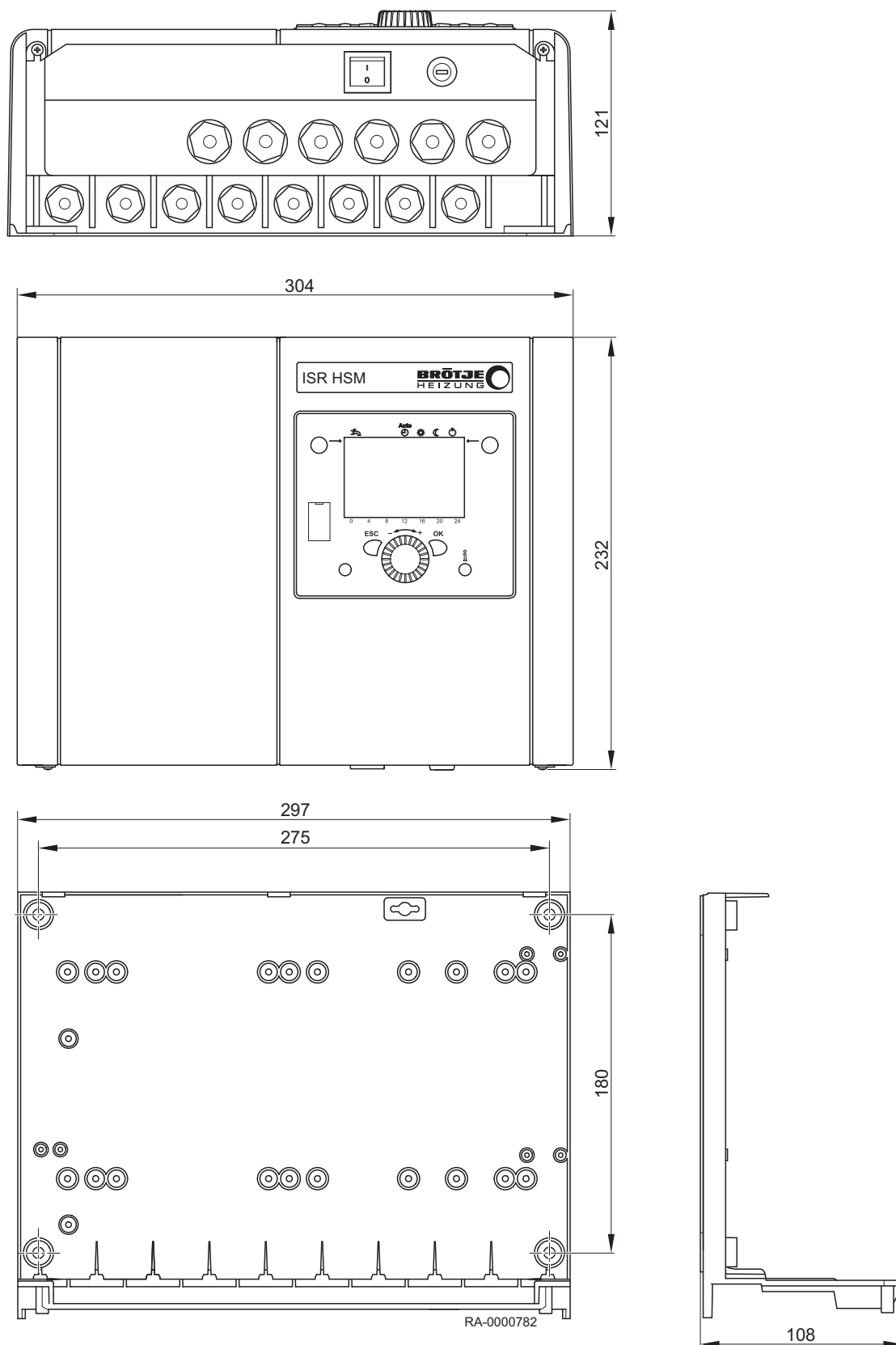
Abb.1 Abmessungen
