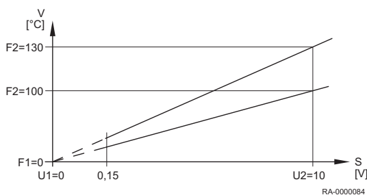
Abb.33 Beispiel für Wärmeanforderung 10 V
