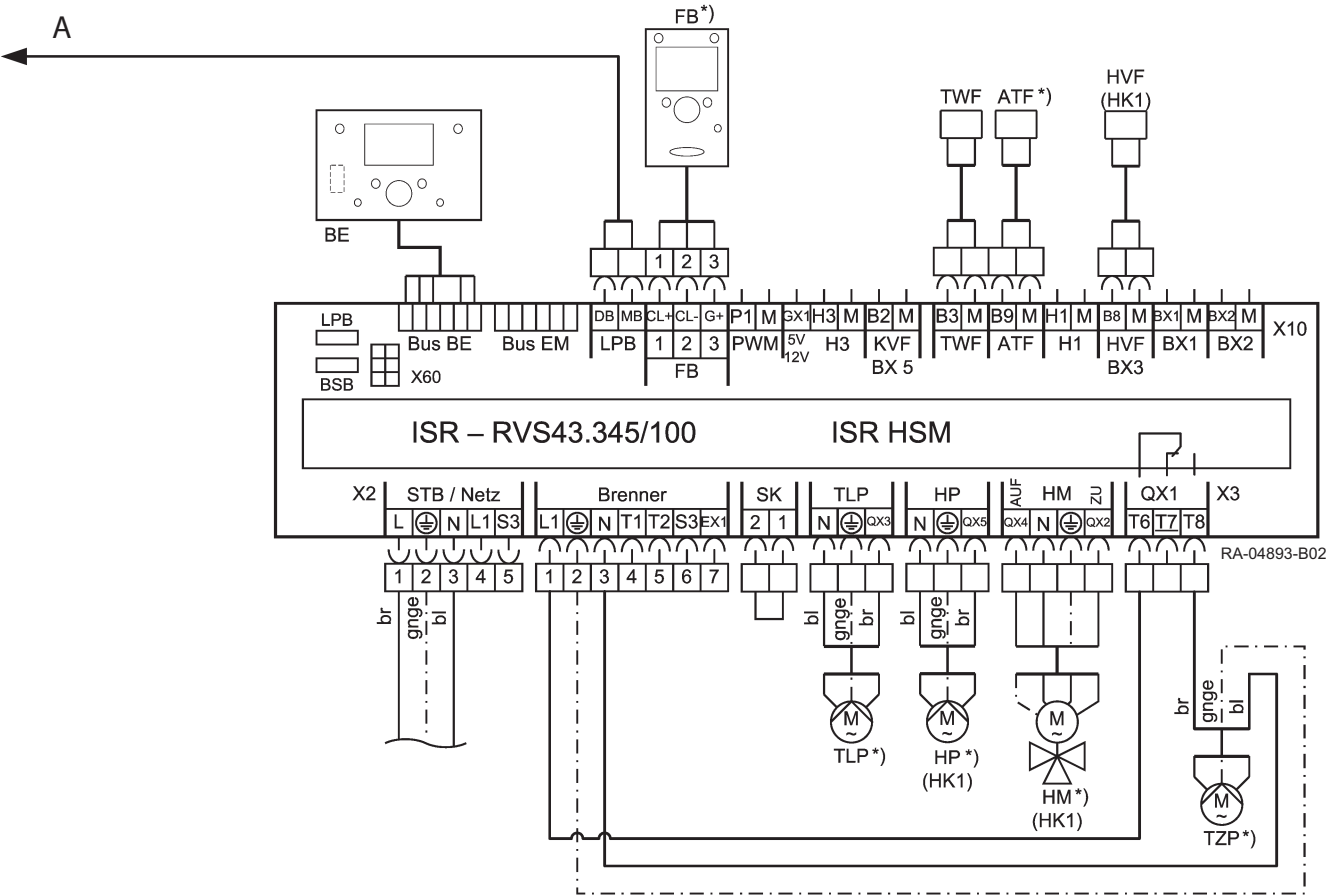
Abb.7 Anschlussplan
