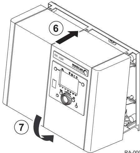
Abb.14 Schließen des Gehäuses
