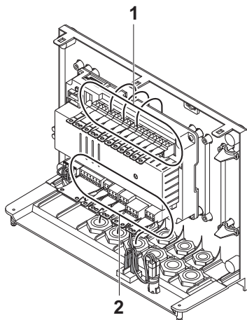
Abb.15 Verlegen der Leitungen im Gehäuse
