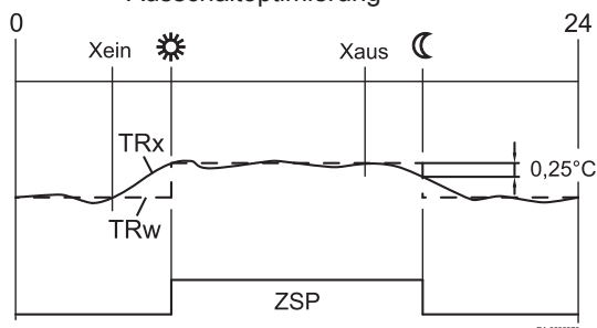
Abb.21 Einschalt- und Ausschaltoptimierung
