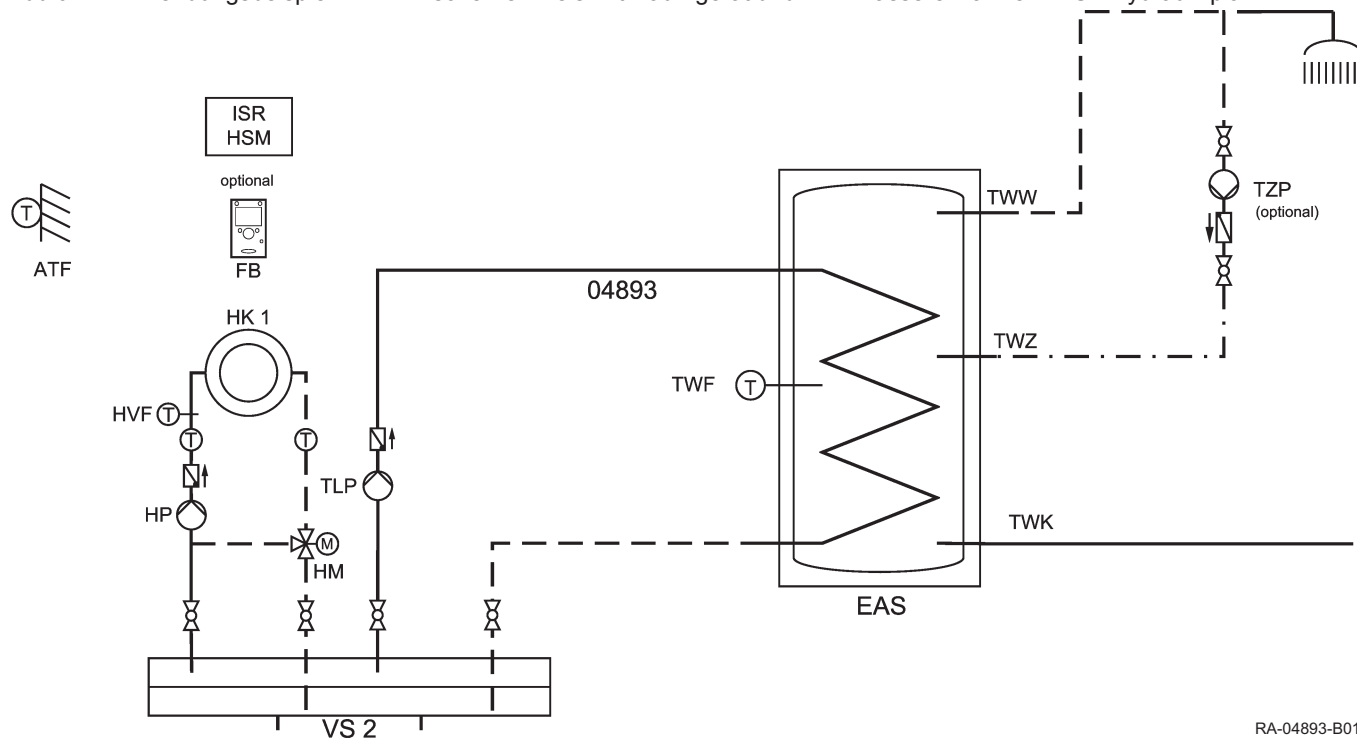
Abb.6 Anwendungsbeispiel 1: Ein Mischerheizkreis mit Raumgerät und Trinkwassererwärmer EAS - Hydraulikplan
