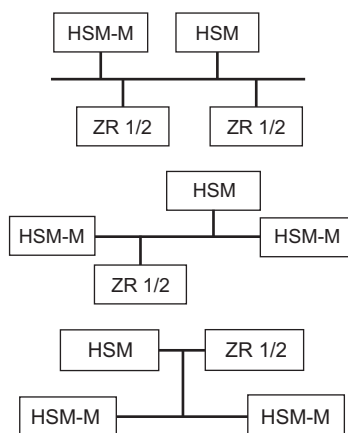
Abb.16 Anschlussmöglichkeiten
