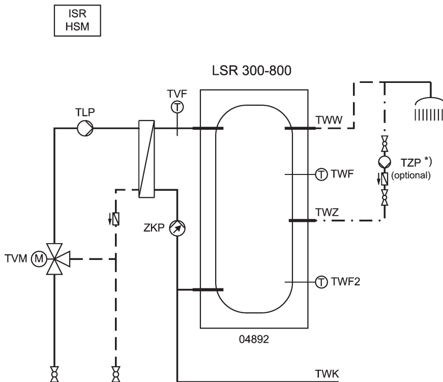
Abb.10 Anwendungsbeispiel 3: Trinkwasser-Speicherladesystem LSR 300-800 inkl. Vorregler - Hydraulikplan
