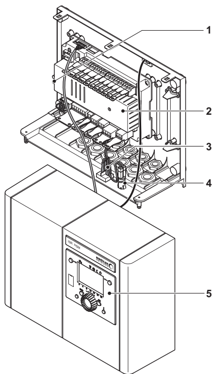
Abb.3 Übersicht HSM
