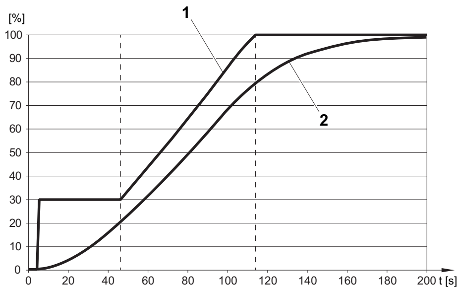
Abb.26 Abhängigkeit Pumpendrehzahl/Erzeugerleistung
