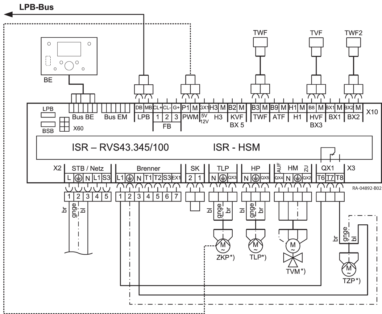
Abb.11 Anschlussplan
