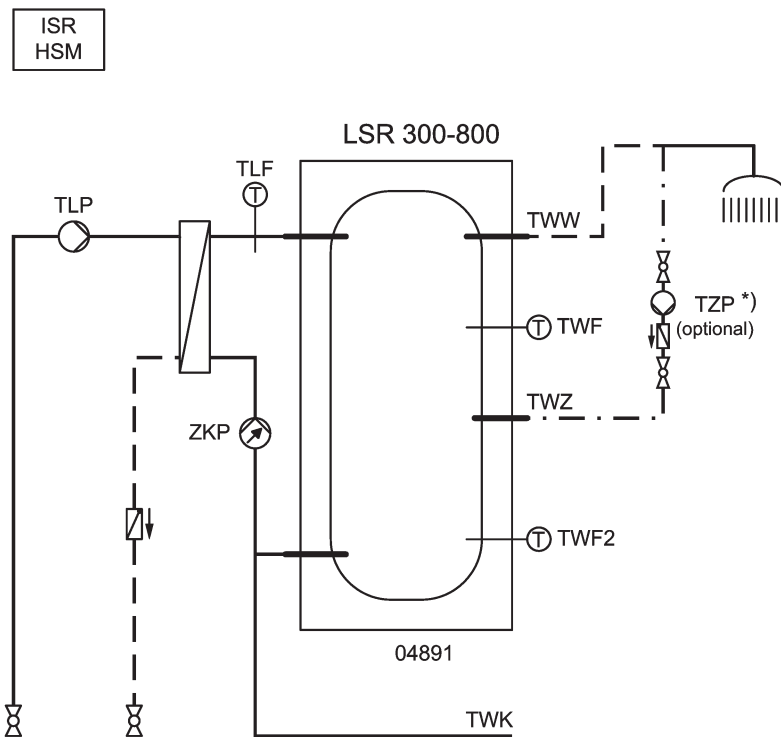
Abb.8 Anwendungsbeispiel 2: Trinkwasser-Speicherrlatesystem LSR 300-800 - Hydraulikplan
