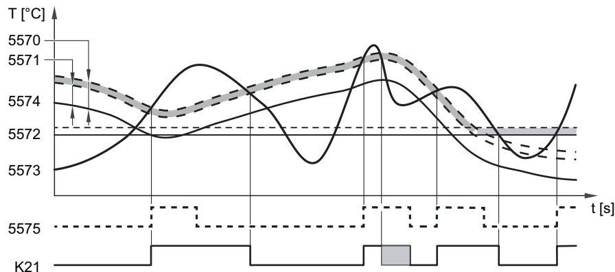
Abb.31 Nutzungsvariante Differenztemperaturregler
