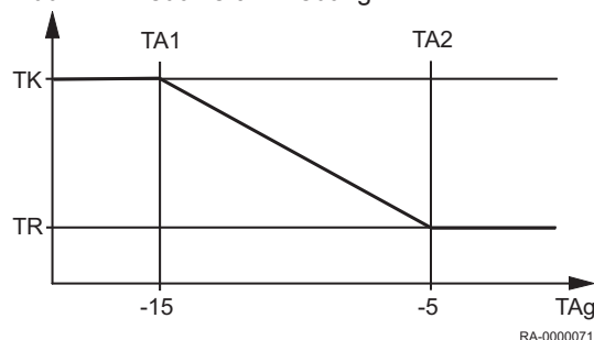
Abb.22 Reduziert-Anhebung
