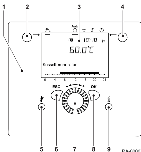
Abb.4 Bedienelemente
