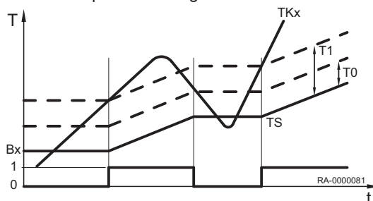
Abb.28 Speicherladung
