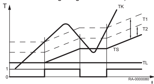
Abb.27 Laderegelung /schematisch)
