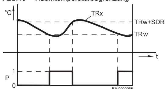
Abb.19 Raumtemperaturbegrenzung
