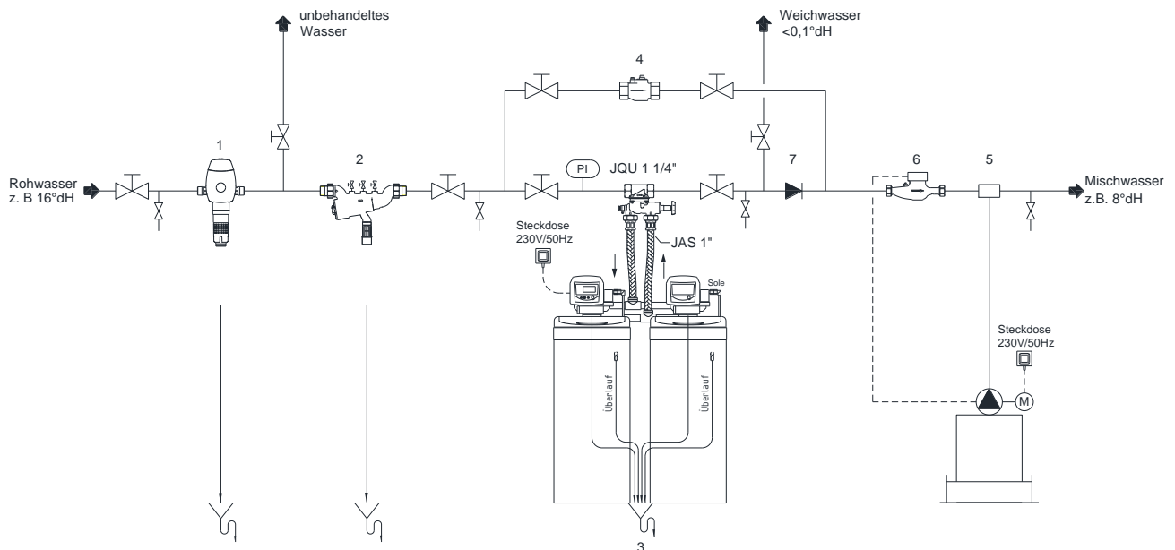
Abb. 4: Installationsbeispiel
