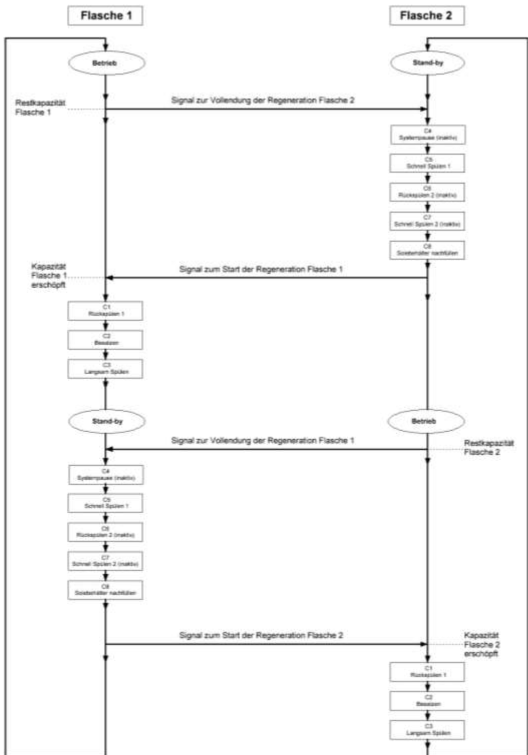
Abb. 2: Schematischer Betriebsablauf
