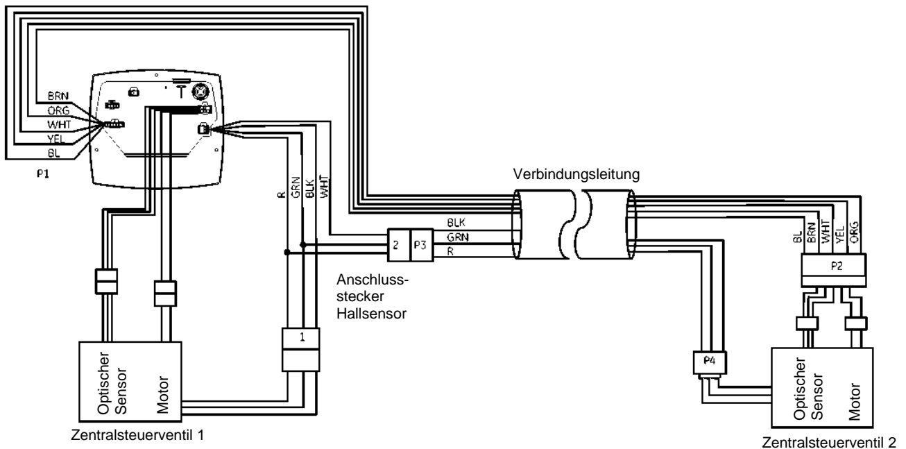
Abb. 5: Anschlussschema Verbindung Zentralsteuerventil 1+2
