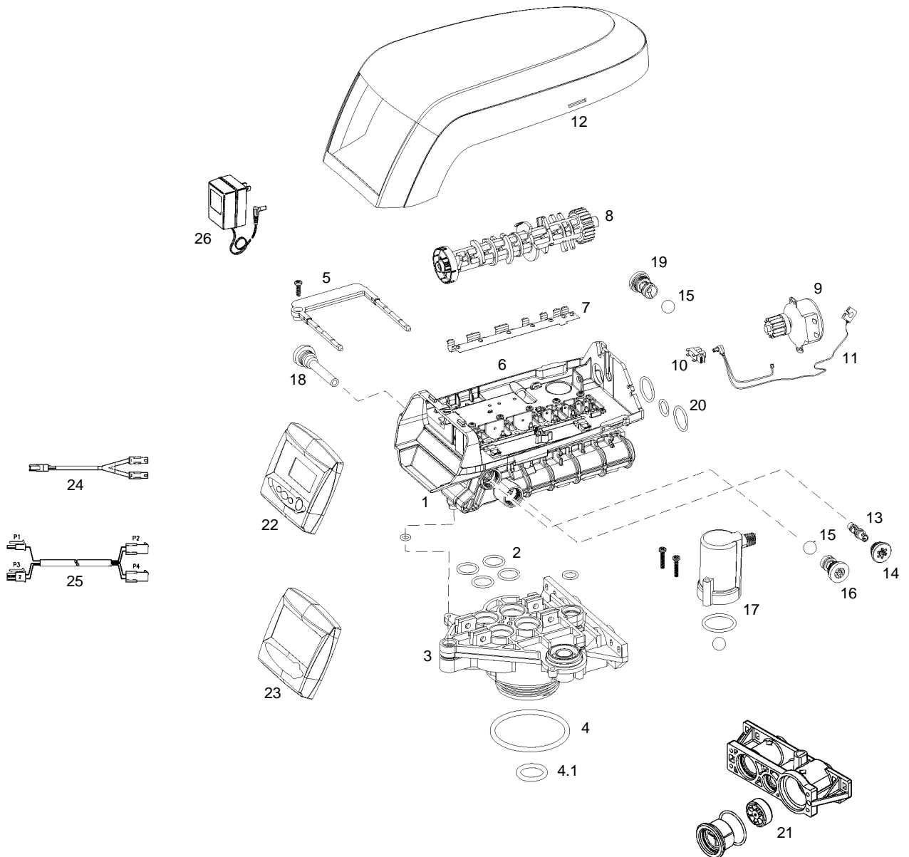
Abb. 13: Explosionszeichnung Zentralsteuerventil
