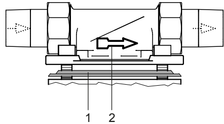
Abb. 2: Einbaudrehflansch
