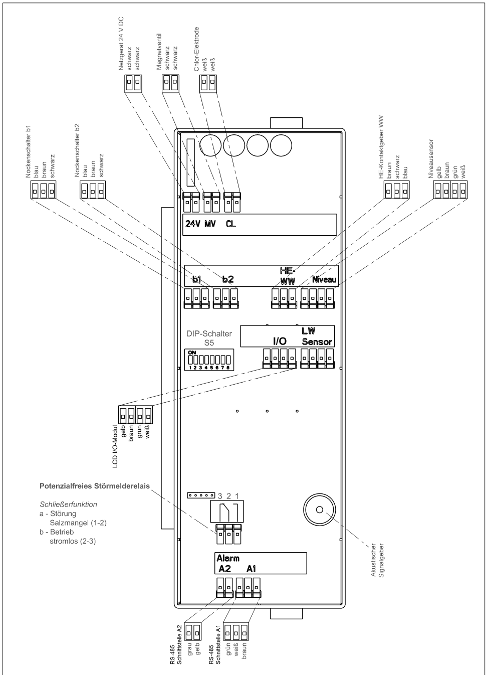
Abb. 8: Elektronische Steuerung mit Störmelderelais
