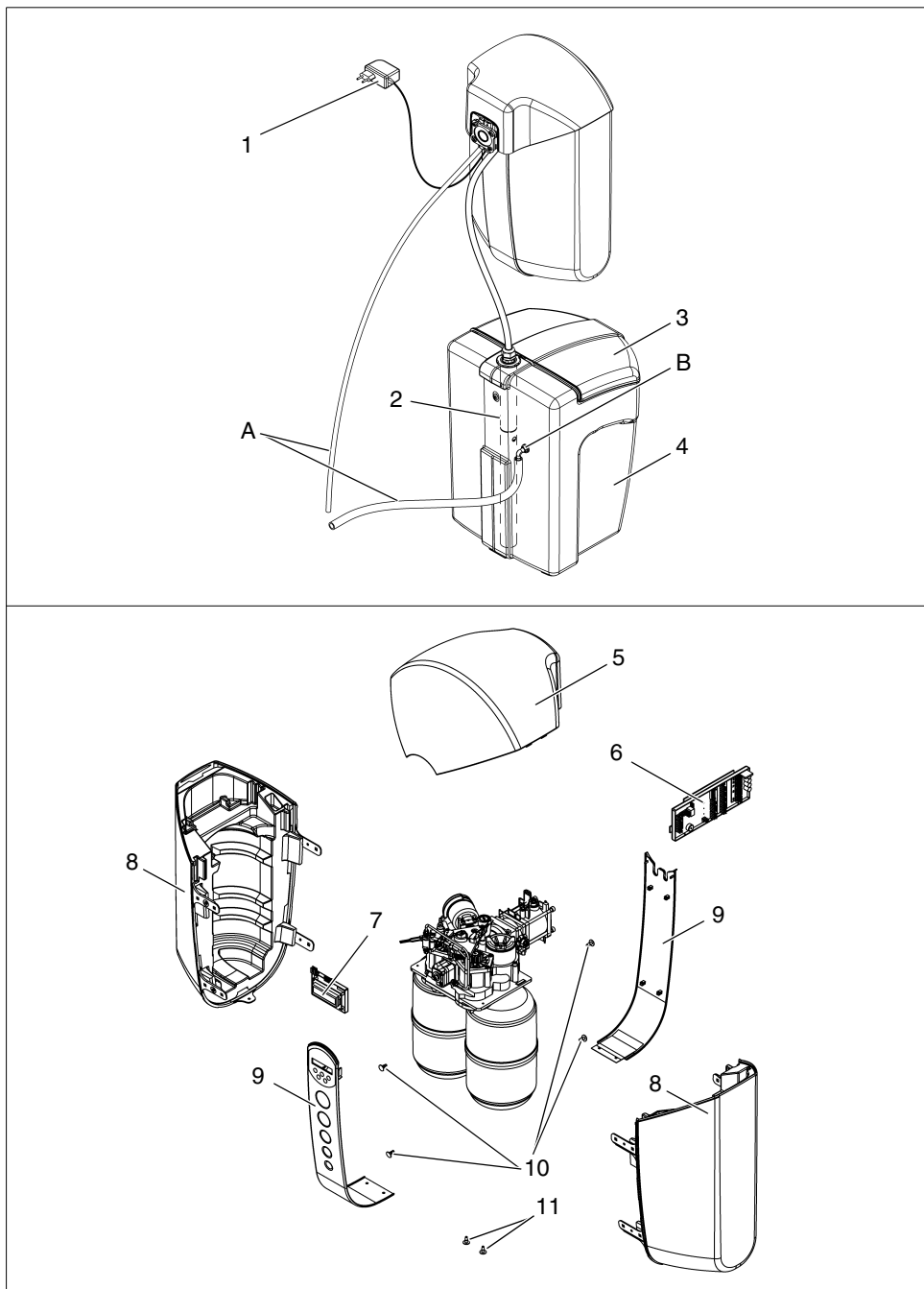
Abb. 9: Ersatzteile JUDO SOFTwell MEGA
