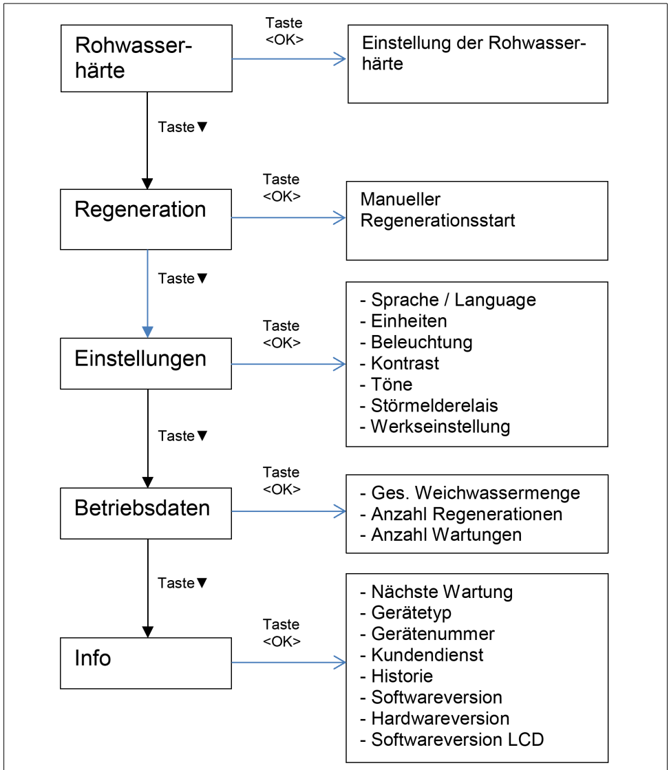
Abb. 7: Menüstruktur
