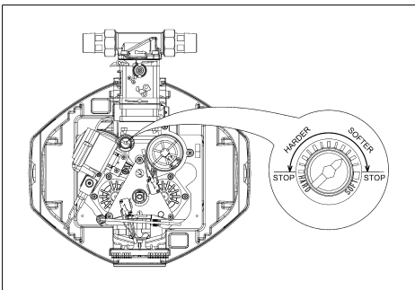
Abb. 6: Einstellen der Verschneidung
