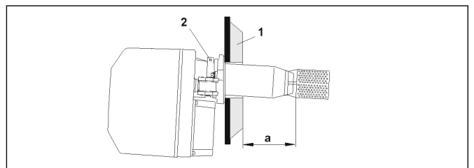
Abb. 3.9: Eintauchtiefe mit Rezirkulationsaufsatz
