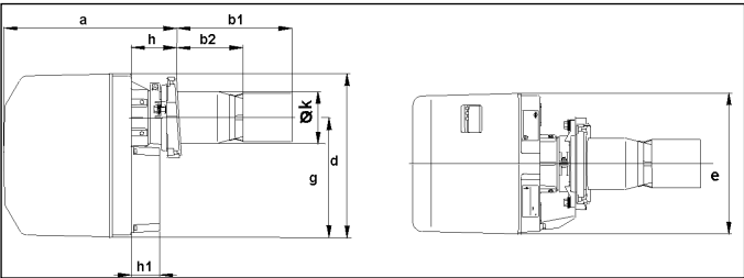
Abb. 5.3: Brennermaße mit Rezirkulationsaufsatz
