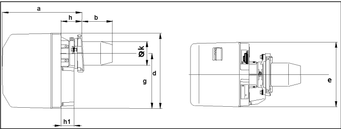
Abb. 5.2: Brennermaße ohne Rezirkulationsaufsatz
