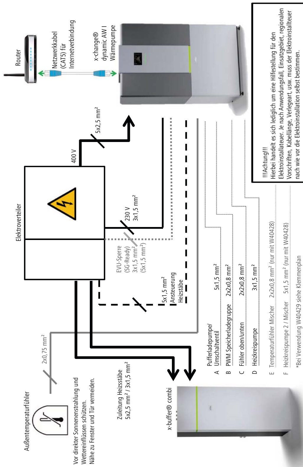
Abb. 42: Elektroinstallationsplan mit x-change® dynamic AW I Luft/Wasser-Wärmepumpe
