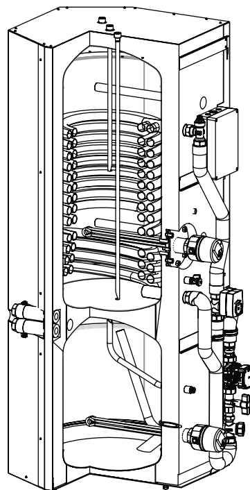
Abb. 1: Schnittdarstellung
