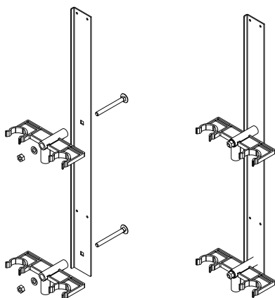
Abb. 16: Montage Halteklammern
