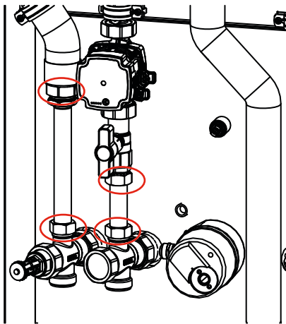
Abb. 22: Demontage Rohre
