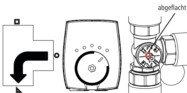
Abb. 32: Stellung Umschaltventil bei Beladung Pufferspeicher
