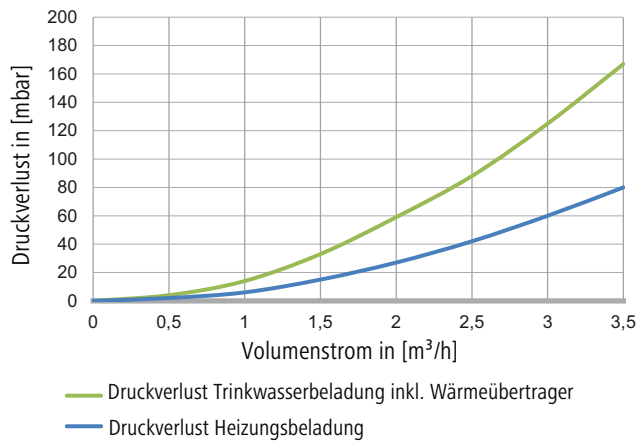
Abb. 36: Druckverlustkennlinie Speicherkombination
