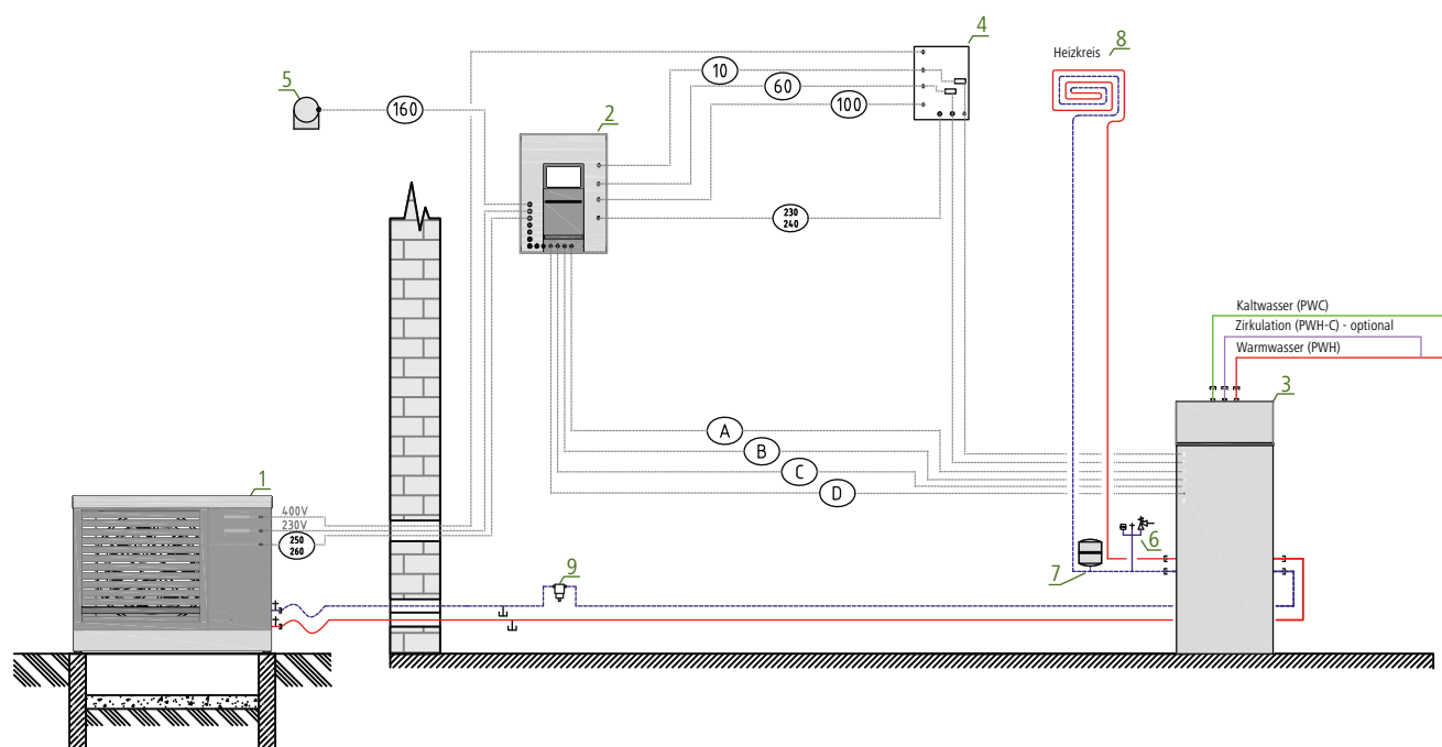
Abb. 39: Hydraulikschema 1 - ein Heizkreis ungemischt
