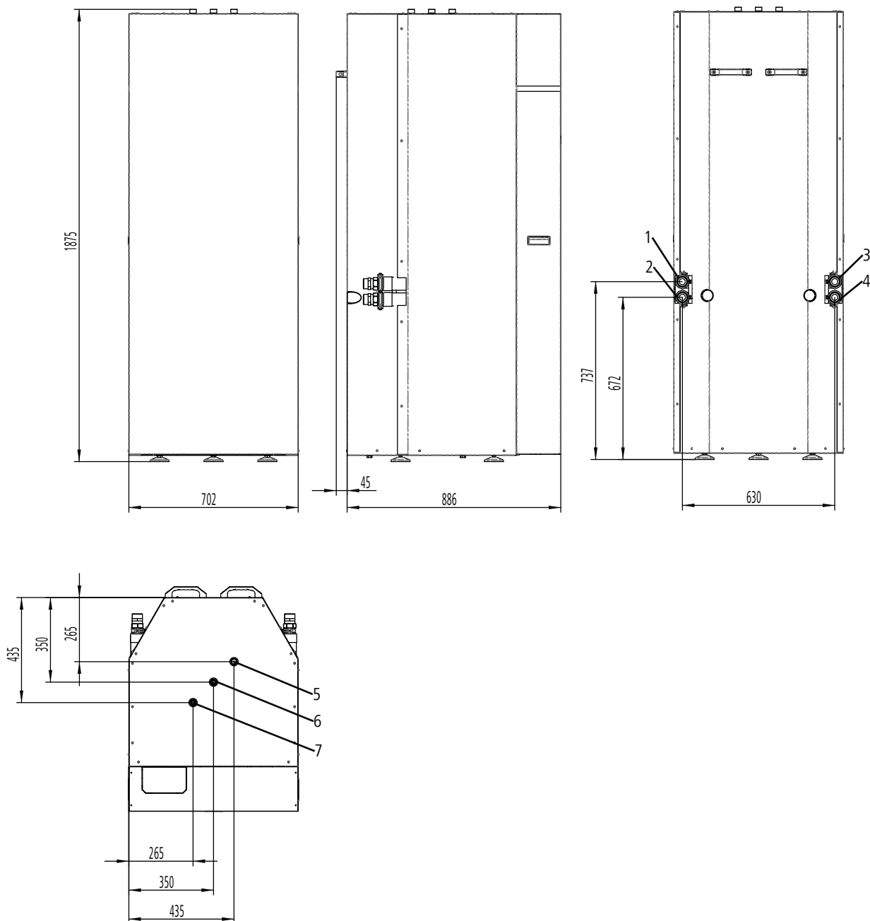
Abb. 37: Abmessungen Speicherkombination
