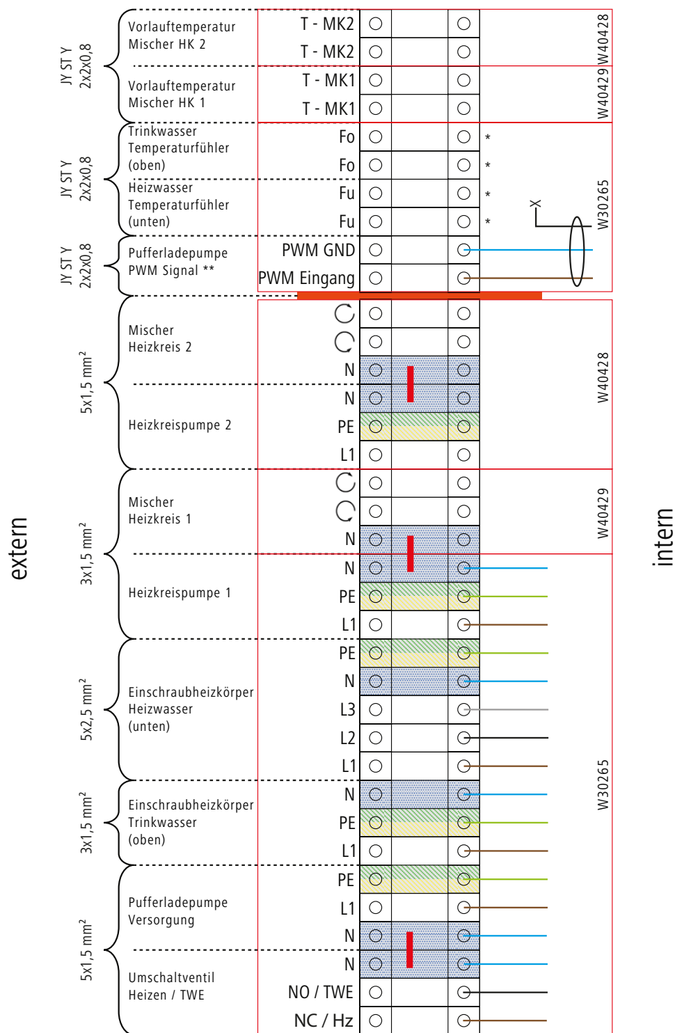
Abb. 46: Klemmenplan Speicherkombination inklusive vollständigem Zubehör (W40428 + W40429)
