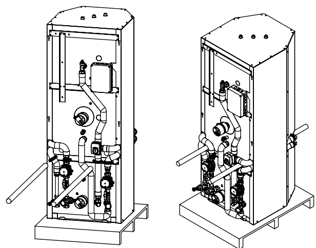
Abb. 5: Rohre in Aussparungen für Tragehilfe
