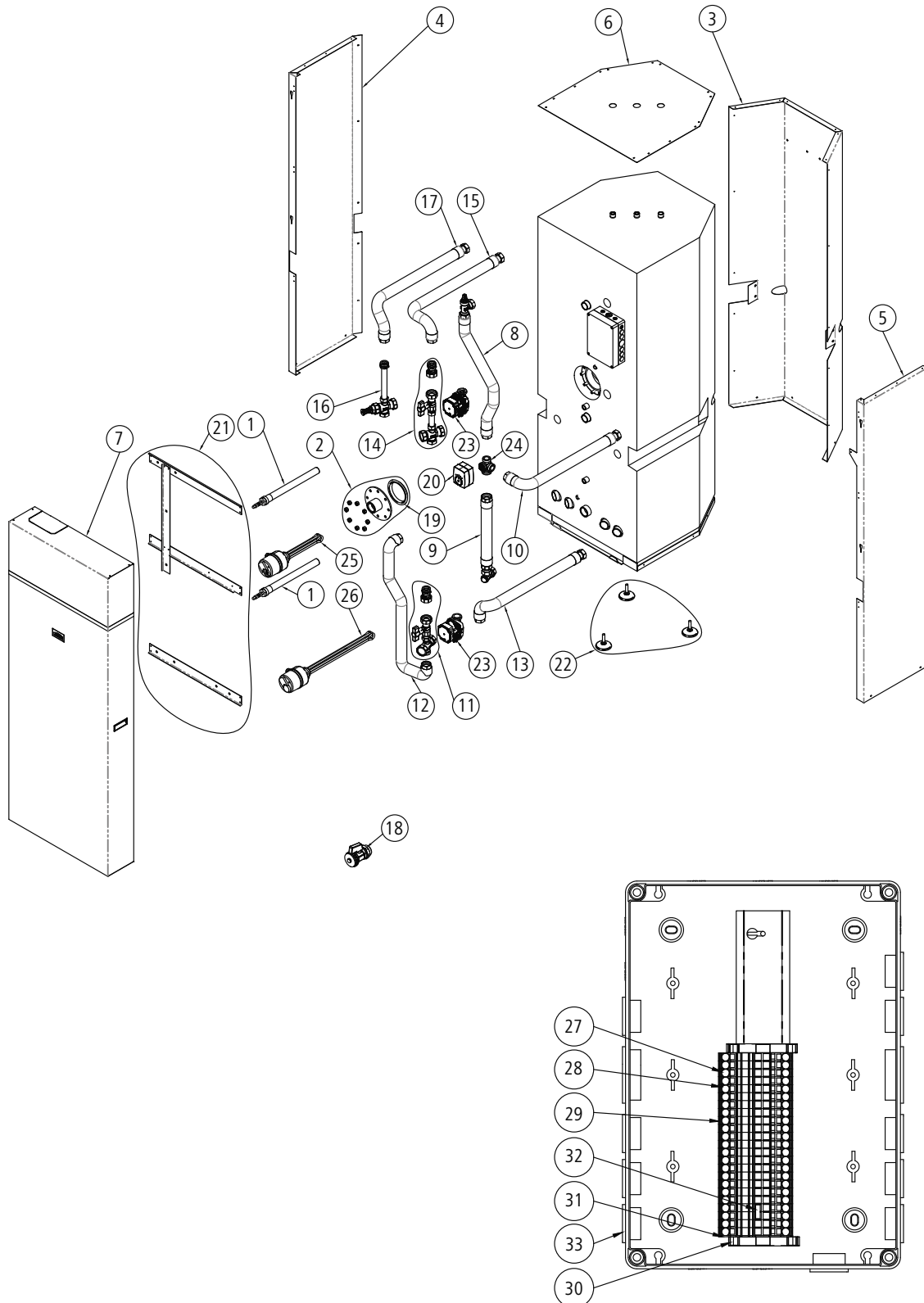
Abb. 38: Ersatzteile
