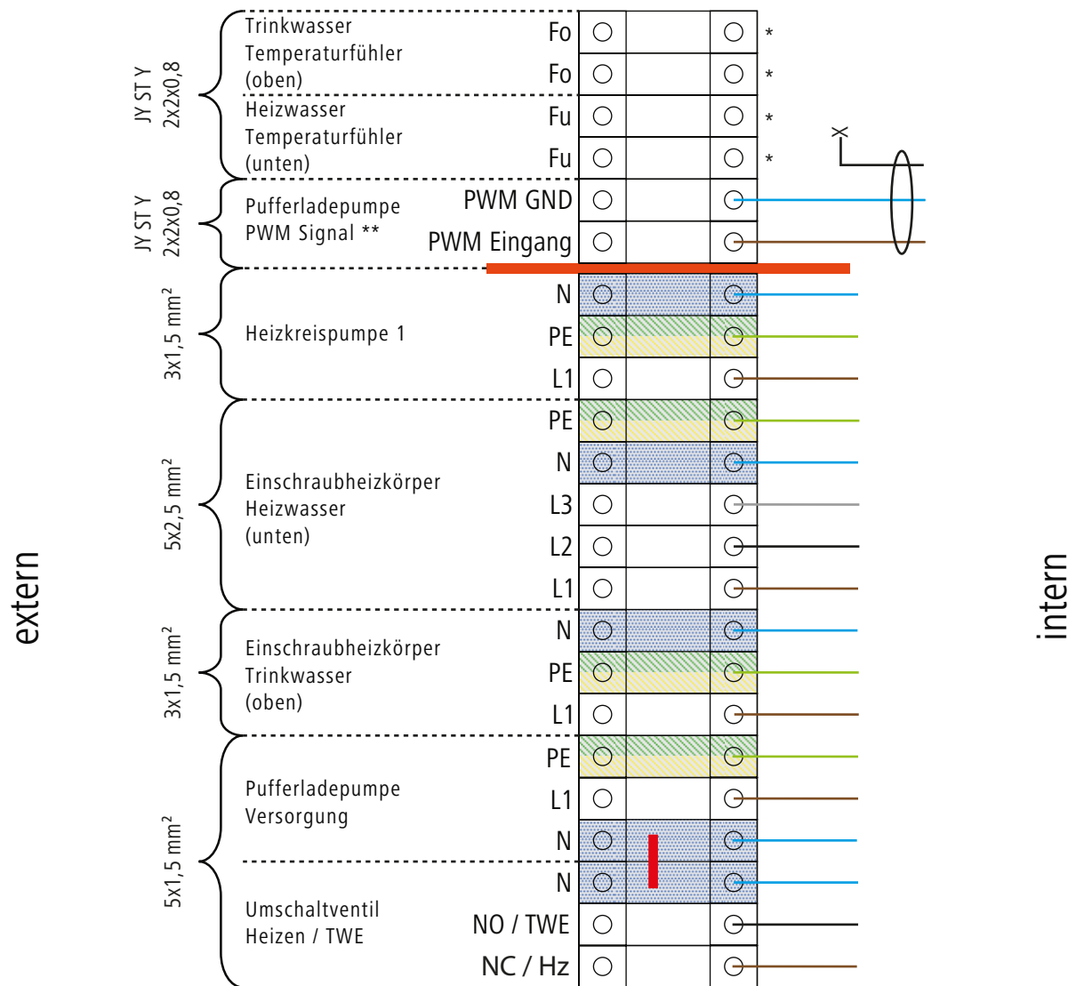
Abb. 44: Klemmenplan Speicherkombination ohne Zubehör
