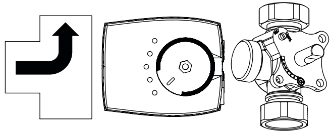
Abb. 25: Stellung 3-Wege-Mischer bei Durchfluss 100% Durchfluss
