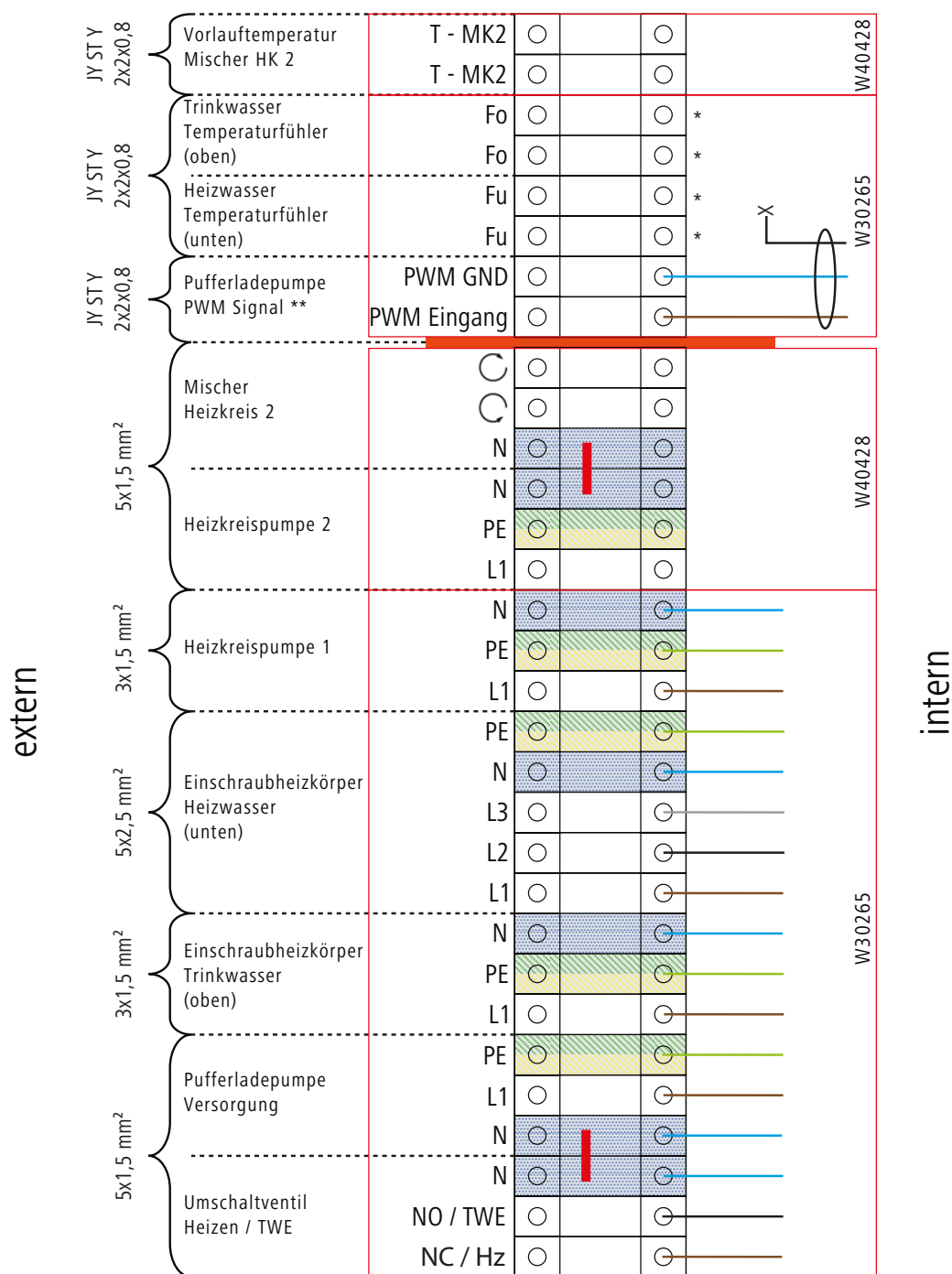
Abb. 45: Klemmenplan Speicherkombination mit Zubehör W40428
