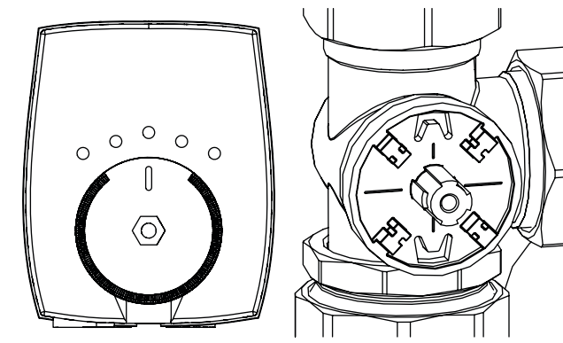
Abb. 31: Stellung Umschaltventil bei Beladung Trinkwasserspeicher
