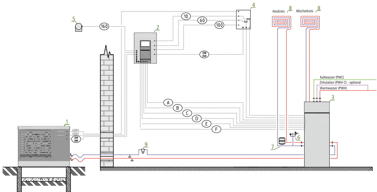
Abb. 40: Hydraulikschema 2 - ein Heizkreis ungemischt und ein Heizkreis gemischt
