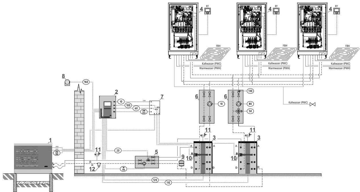
Abb. 20: 5-Leiter Wohnungsstation DYA-CPU-CPU-WST-01
