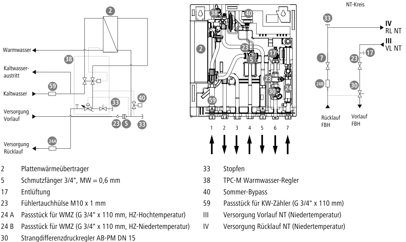
Abb. 3: Komponenten der x-net Wohnungsstation 5-Leiter
