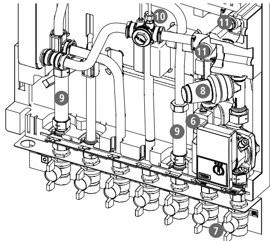
Abb. 8: Komponentenübersicht 6 - 11
