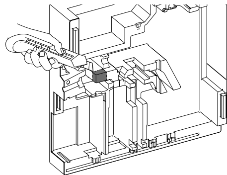
Abb. 11: Dämmhaube
