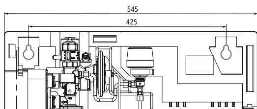
Abb. 5: Montageposition x-net Wohnungsstation
