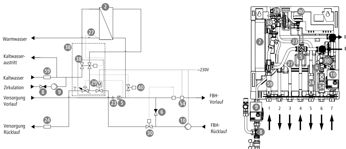
Abb. 2: Komponenten der x-net Wohnungsstation mit gem. HK
