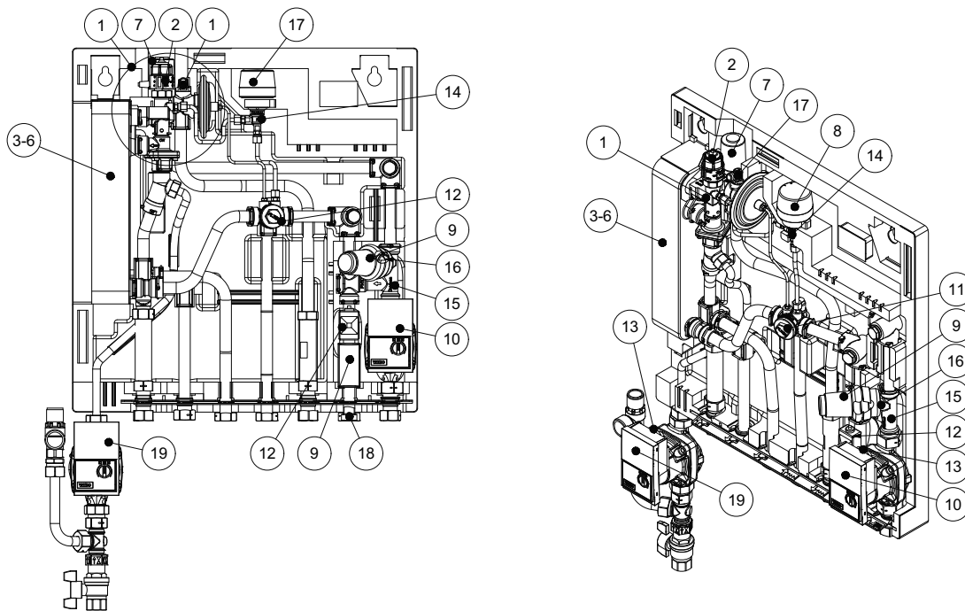
Abb. 18: Übersicht Ersatzteile
