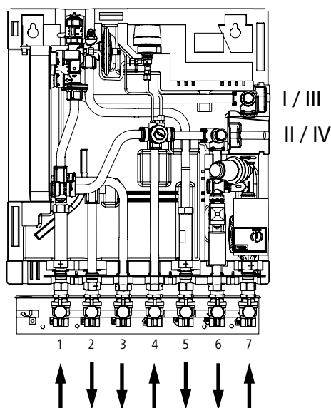
Abb. 4: Anschluss an x-net Wohnungsstation
