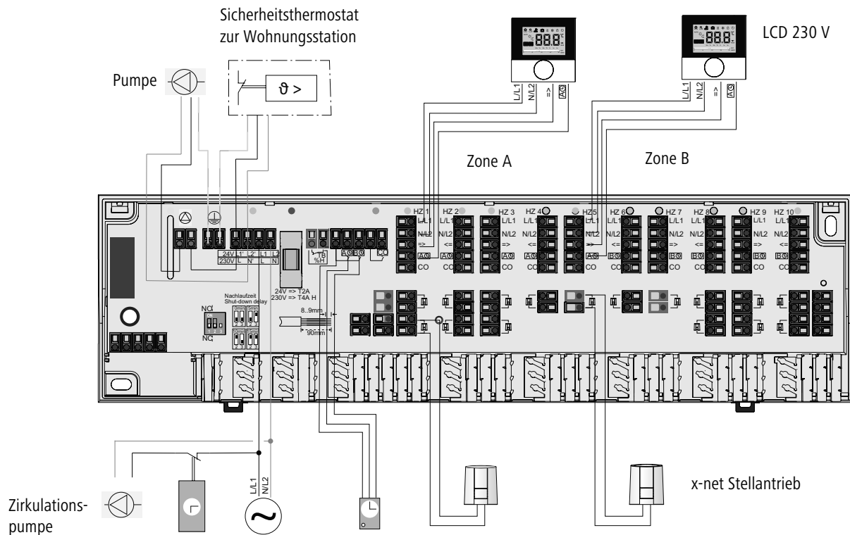
Abb. 6: Schema elektrischer Anschluss
