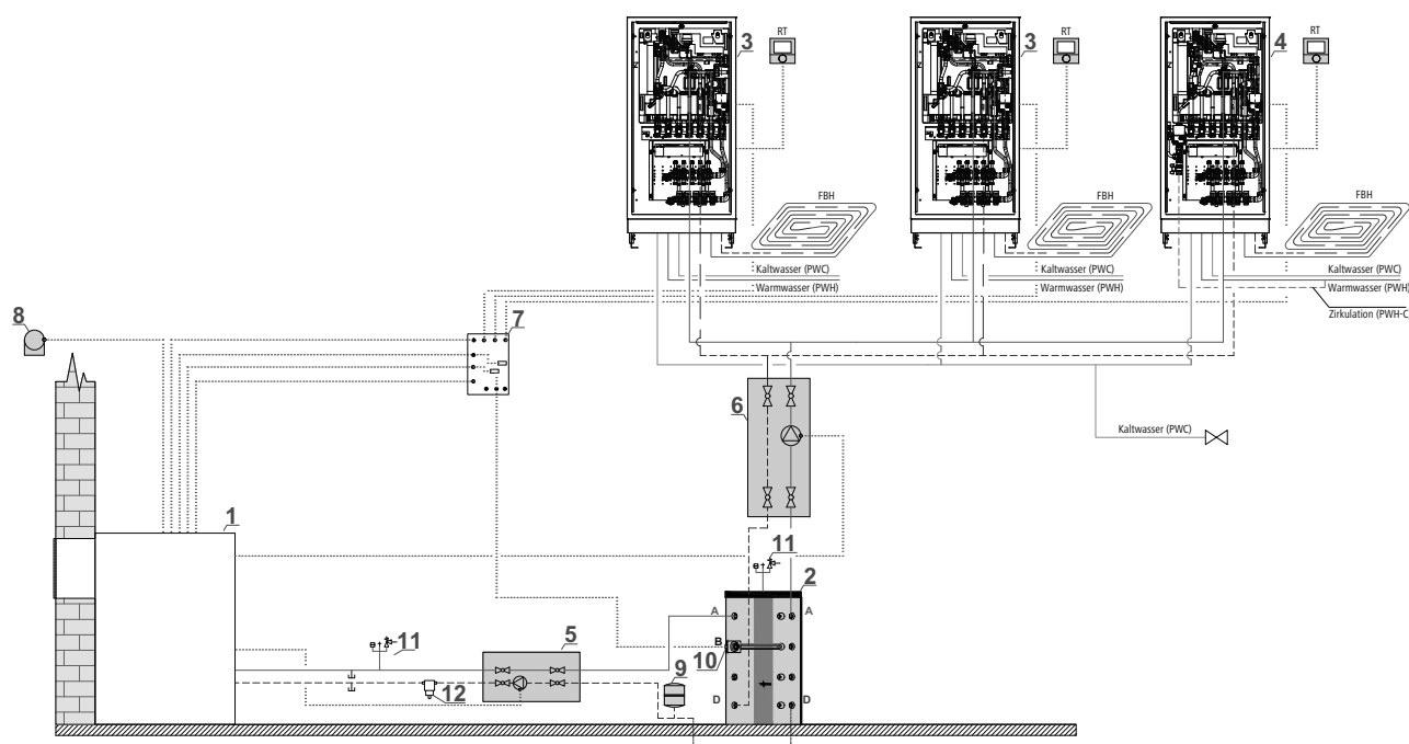
Abb. 19: 3-Leiter Wohnungsstation
