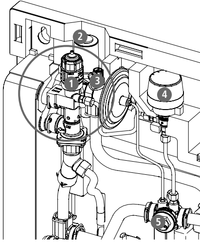
Abb. 7: Komponentenübersicht 1 - 5
