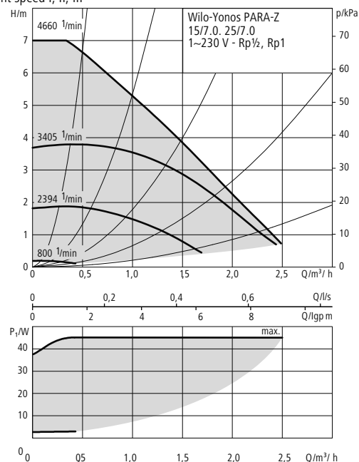
Abb. 14: Pumpendiagramm Zirkulationspumpe
