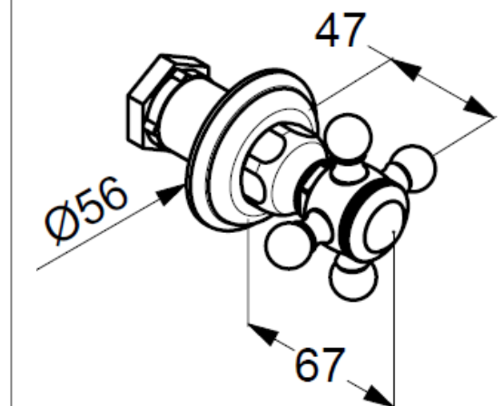
Maßzeichnung
