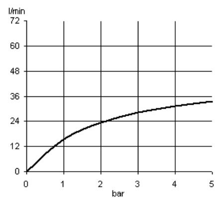
Durchflussdiagramm
