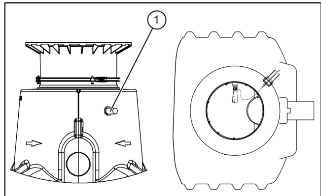
Fig.: Figura esemplificativa per tubo per cavi sul serbatoio
