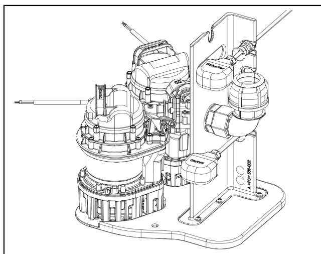
Fig. 1: Esempio di adattatore filettato
