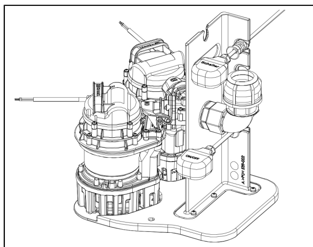
Afb. 1: Voorbeeld van schroefadapters
