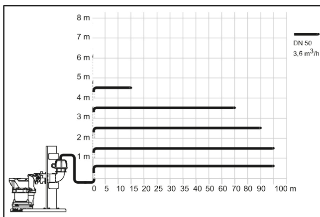
Fig.: Courbe de rendement Retrofit 500
