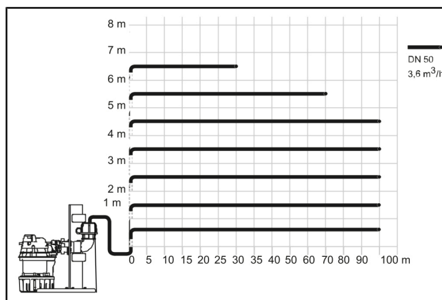
Rys.: Wykres wydajności Retrofit 1000
