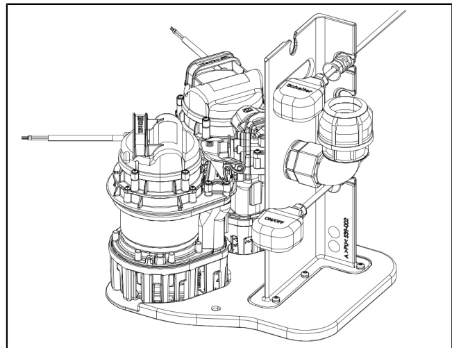
Rys. 1: Przykład z adapterem gwintowym
