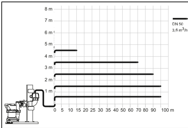
Afb.: Capaciteitsdiagram Retrofit 500
