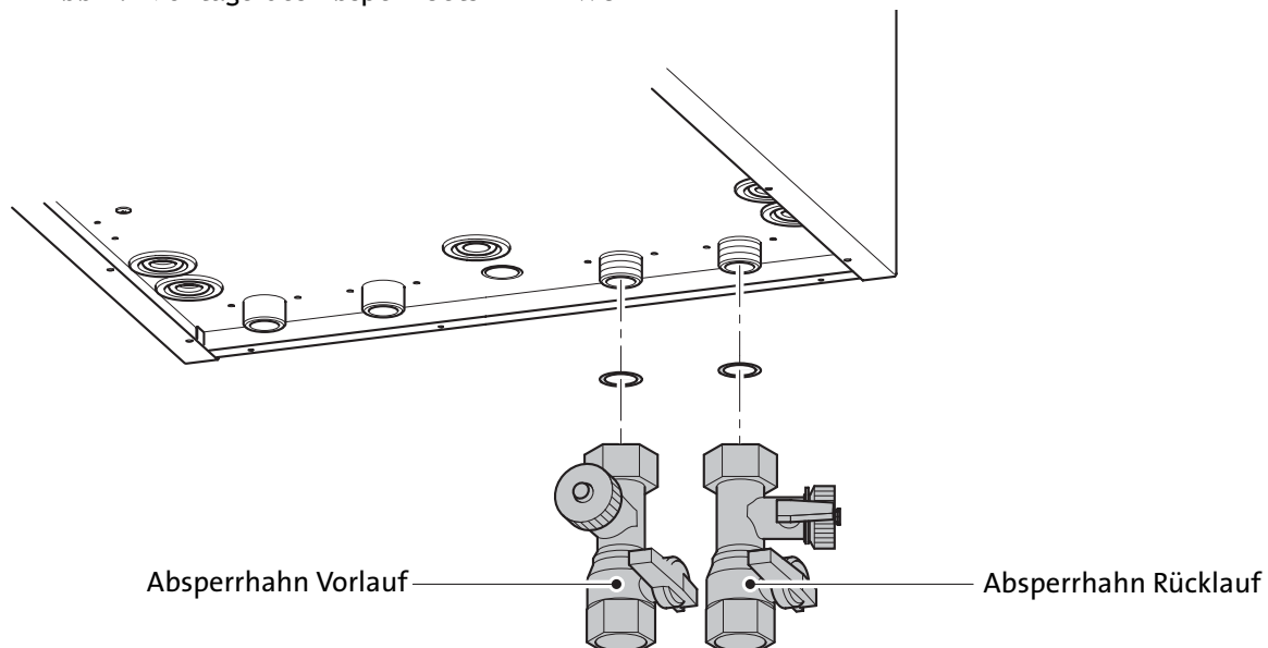
Abb 1: Montage des Absperr-Sets ADH 2 WOB
