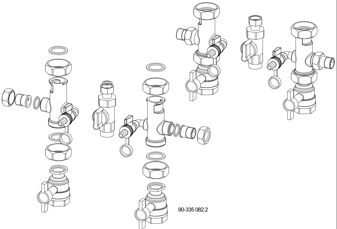
Abb. 1 Montage ADH 1½"
