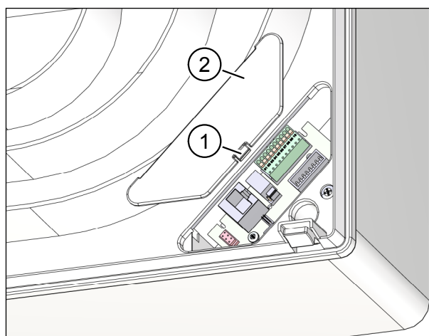
Abb. 3: Netzwerkdeckel abnehmen
