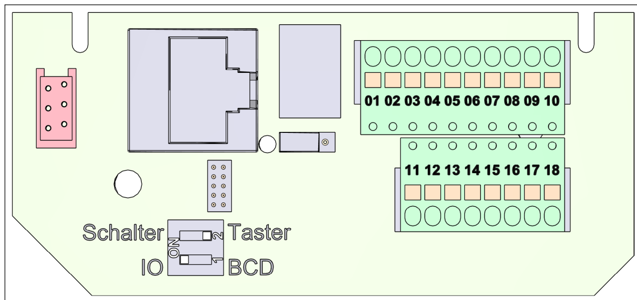
Abb. 15: Platine im Lüftungsgerät M-WRG-S/Z-KNX (-F, -FC)
