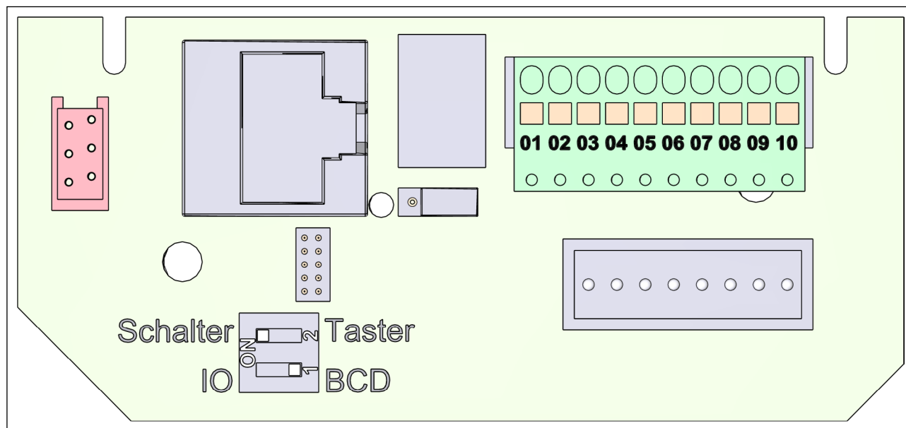
Abb. 6: Platine im Lüftungsgerät M-WRG-S/Z-24
