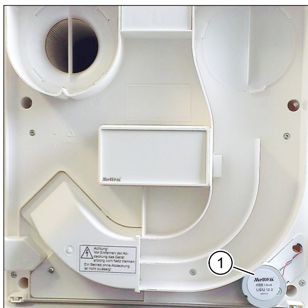
Abb. 16: KNX-Schnittstelle
