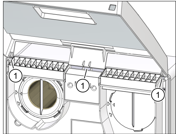
Abb. 5: Deckeldrehpunkte
