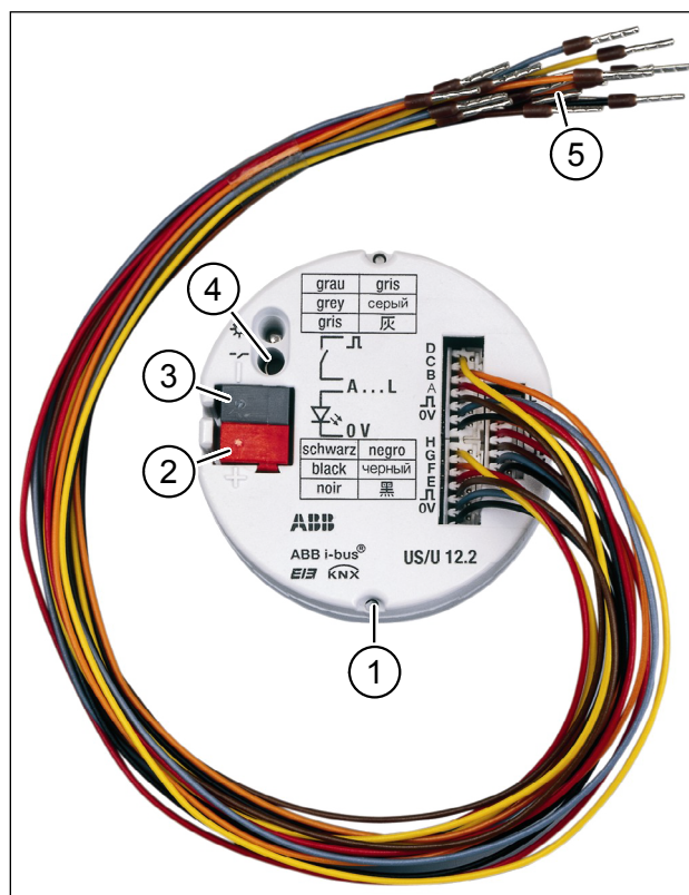
Abb. 14: KNX-Schnittstelle ABB US/U 12.2
