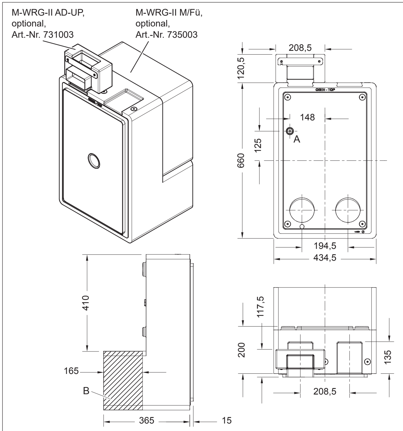
Abb. 7: Abmessungen des Montagesets in Millimeter
