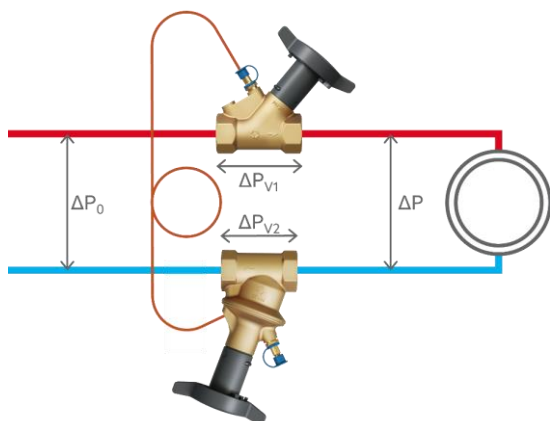
Systemdarstellung
