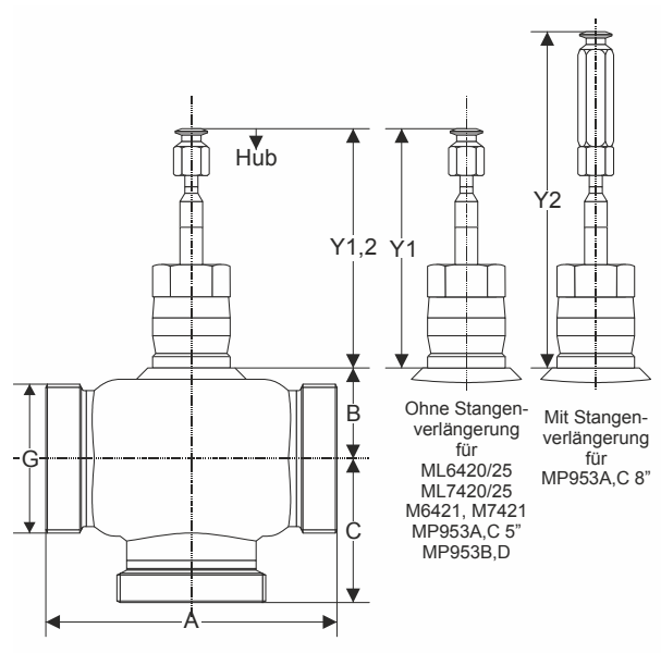
Abb. 2. Abmessungen, V5013E
