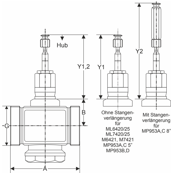
Abb. 1. Abmessungen, V5011E
