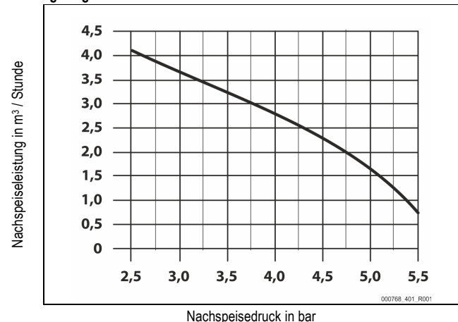
Leistungsdiagramm
