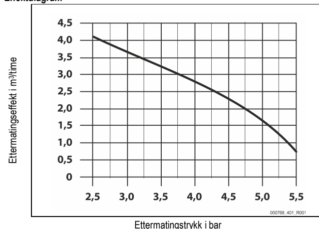
Effektdiagram
