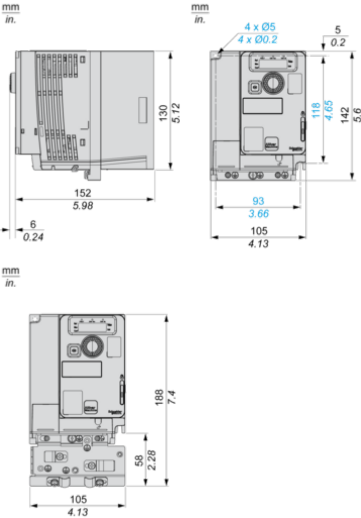
Rechtsseitige Ansicht, Vorderansicht und Vorderansicht mit EMV-Platte
