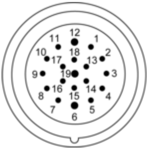
M23-Steckverbinder
