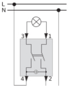
Aus-Kontrollschalter, 2-polig Mxx3x02-0000
