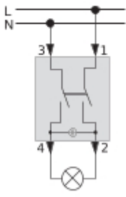
Aus-Kontrollschalter, 2-polig Mxx3x02-0000
