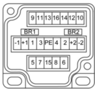
Anschlussklemmen
