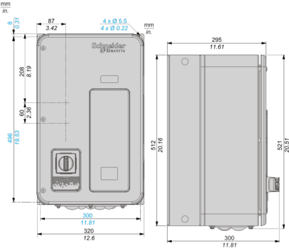
Vorderansicht und linksseitige Ansicht
