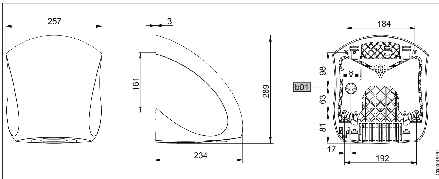
b01 Průchodka el. rozvodů
