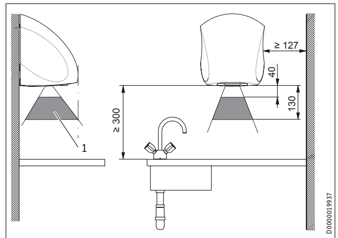
1 Detectiebereik van de infraroodsensor
