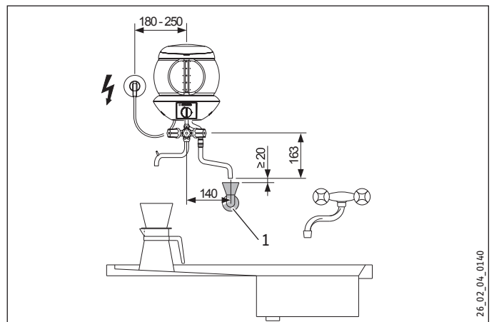
1 Ablauftrichter mit Geruchverschluss
