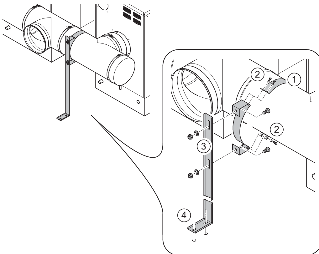
Abb. 1: Entfernen der Abdeckplatte und Montage des Rohrstücks
