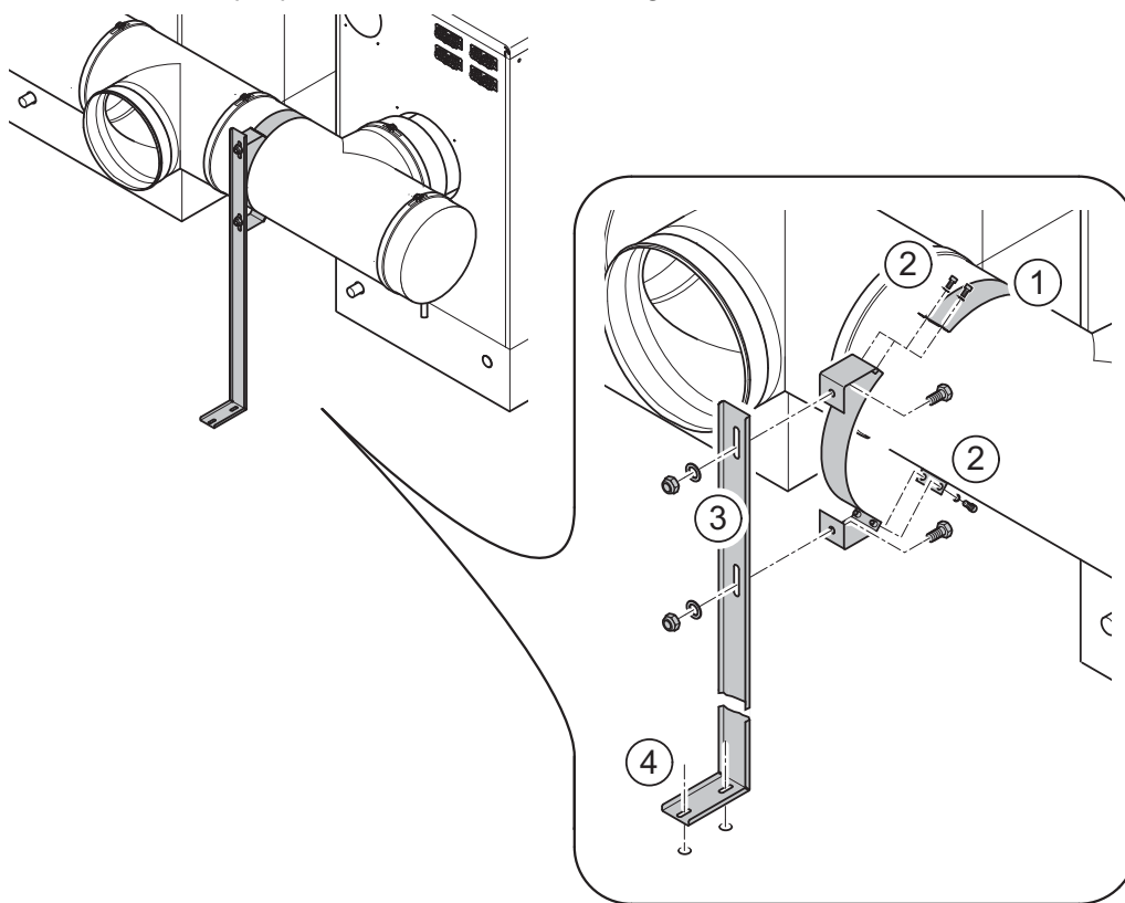
Fig. 1: Enlèvement de la plaque de recouvrement et montage de l'élément tubulaire
